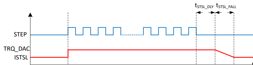
図 7-12. 静止電力節約モード
