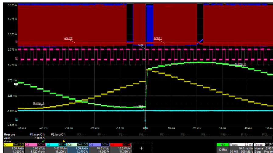
図 7-5. インデクサのリセット
