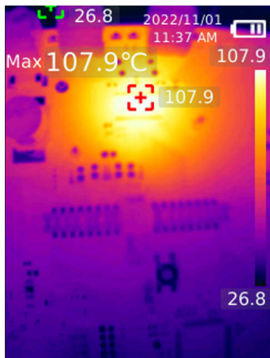
図 8-7. DRV8462、DDW パッケージ、自動トルク・デ ィセーブル
