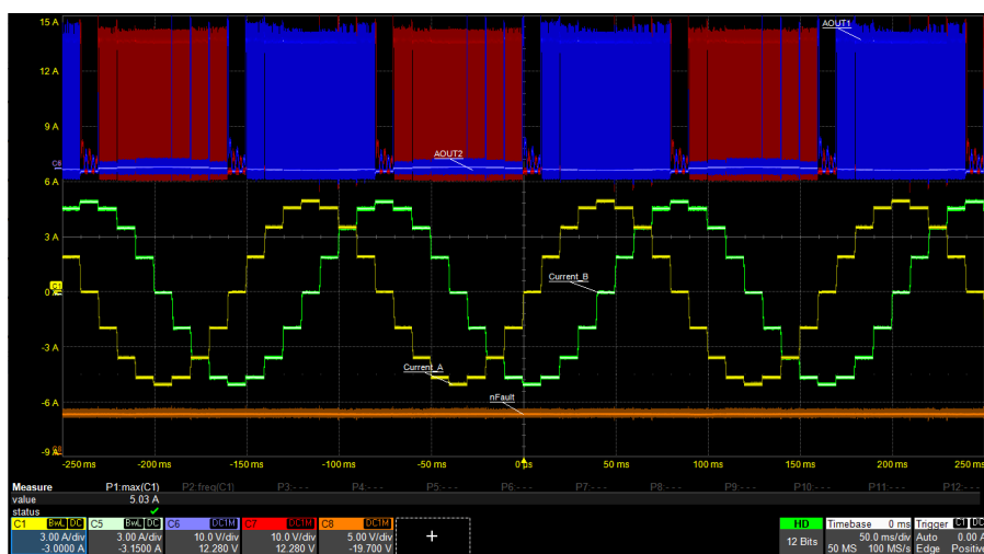
図 8-4. I_{FS} = 5A による 100pps での 1/4 マイクロステッピング
