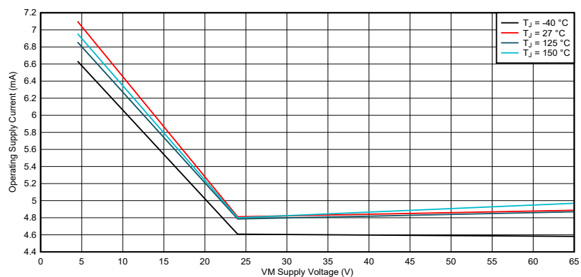
図 6-4. 動作電源電流、VCC = 外部 5V
