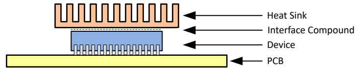
図 9-1. DDV パッケージのヒートシンク
