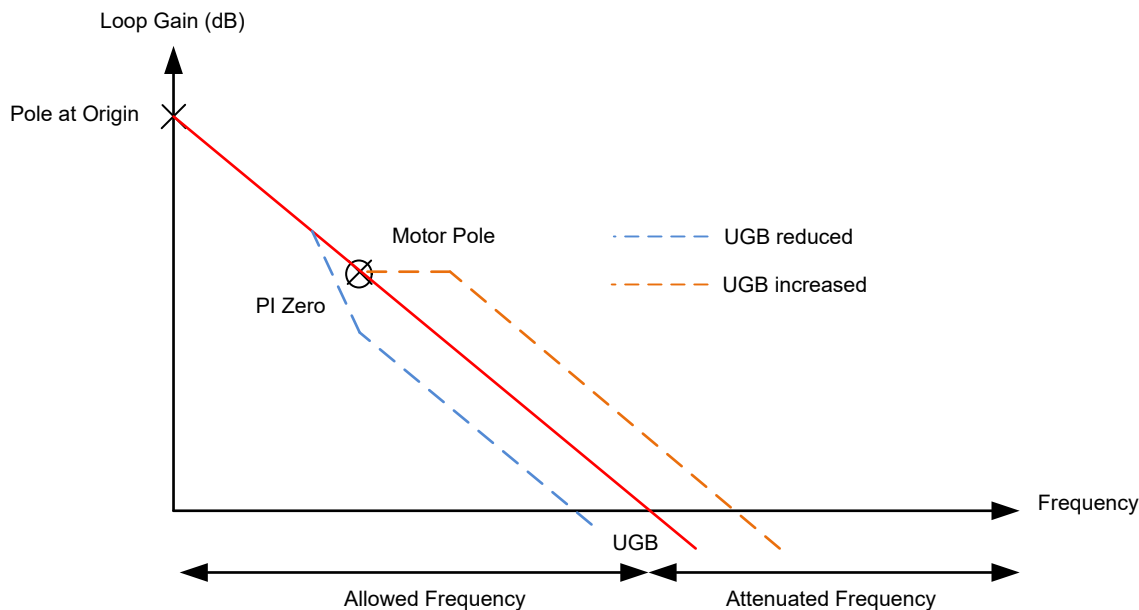
図 7-20. サイレント・ステップ・ゲインと周波数との関係
