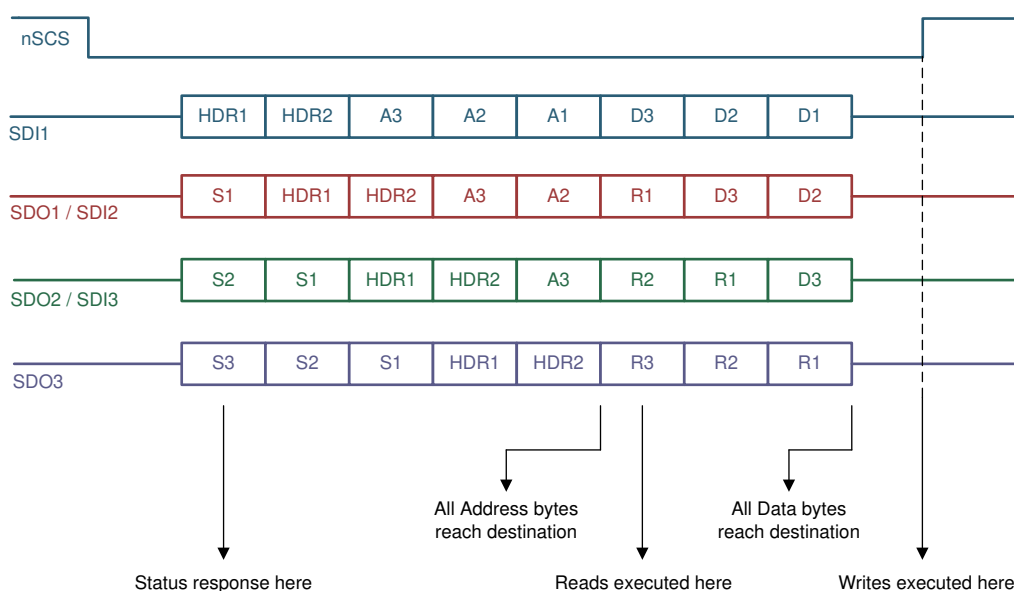
図 7-51. 3 台のデバイスによる SPI フレーム
