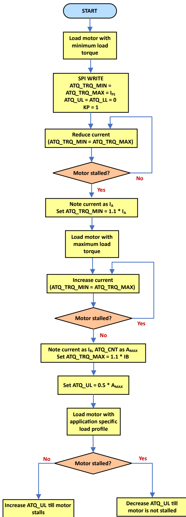
図 7-29. ATQ_TRQ_MIN、ATQ_TRQ_MAX、ATQ_UL、ATQ_LL の選択
