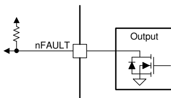
図 7-47. nFAULT ピン
