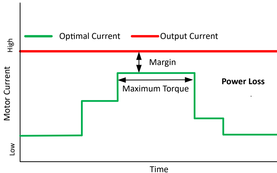
図 7-23. 標準型ステッパ・ドライバによる電力損失
