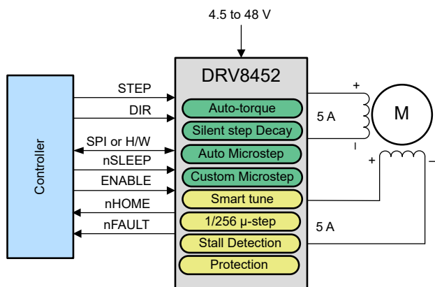
概略回路図
