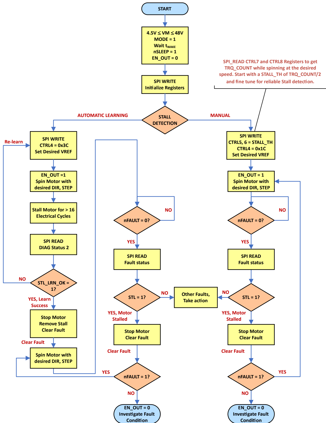
図 7-44. ストール学習フローチャート
