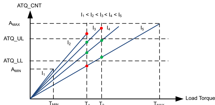
図 7-27. 負荷トルクの間数としての ATQ_CNT
