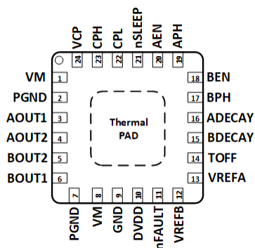
図 5-2. RGE パッケージ 24 ピン VQFN (露出サーマル・パッド付き) 上面図 DRV8434E
