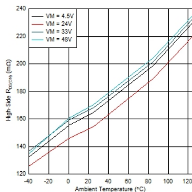
図 6-8. ハイスайд R_{DS(ON)} 温度特性
