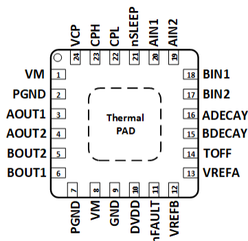
図 5-4. RGE パッケージ 24 ピン VQFN (露出サーマル・パッド付き) 上面図 DRV8434E
