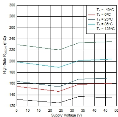
図 6-7. ハイスайд R_{DS(ON)} と電源電圧
