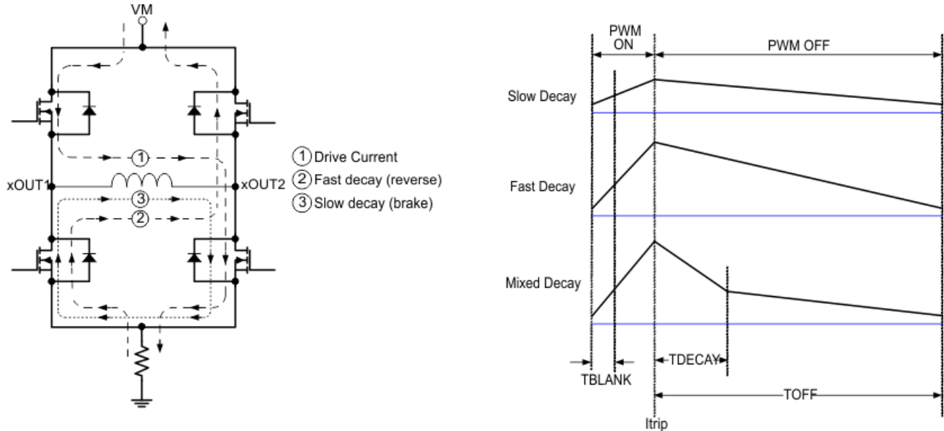
図 7-4. ディケイ・モード
