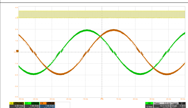
図 8-6. スマート・チューン・ダイナミック・ディレイによる 1/32 マイクロステッピング
