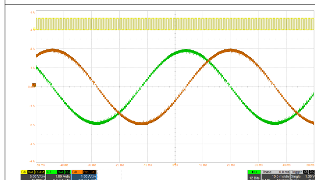
図 8-5. スマート・チューン・リップル・コントロール・ディレイによる 1/32 マイクロステッピング
