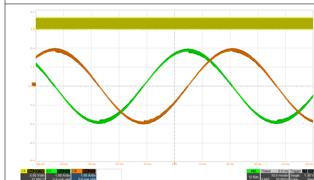
図 8-7. スマート・チューン・リップル・コントロール・ディレイによる 1/256 マイクロステッピング
