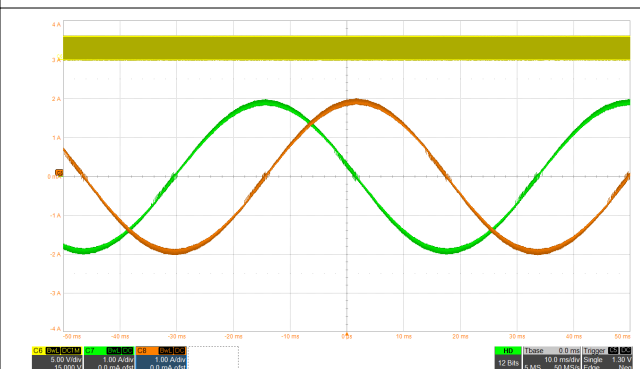
図 8-8. スマート・チューン・ダイナミック・ディレイによる 1/256 マイクロステッピング
