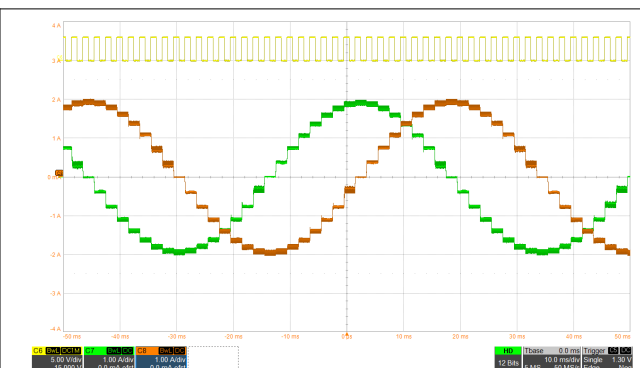
図 8-4. スマート・チューン・ダイナミック・ディレイによる 1/8 マイクロステッピング
