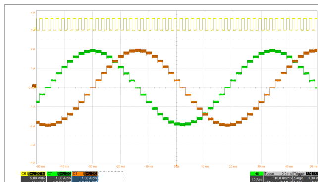
図 8-3. スマート・チューン・リップル・コントロール・ディレイによる 1/8 マイクロステッピング
