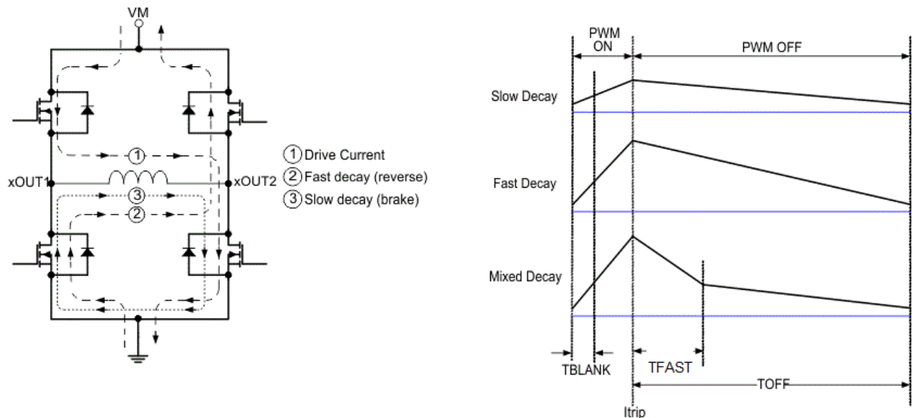
図 7-5. 減衰モード
