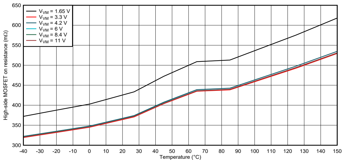
図 7-3. ハイスайд MOSFET オン抵抗
