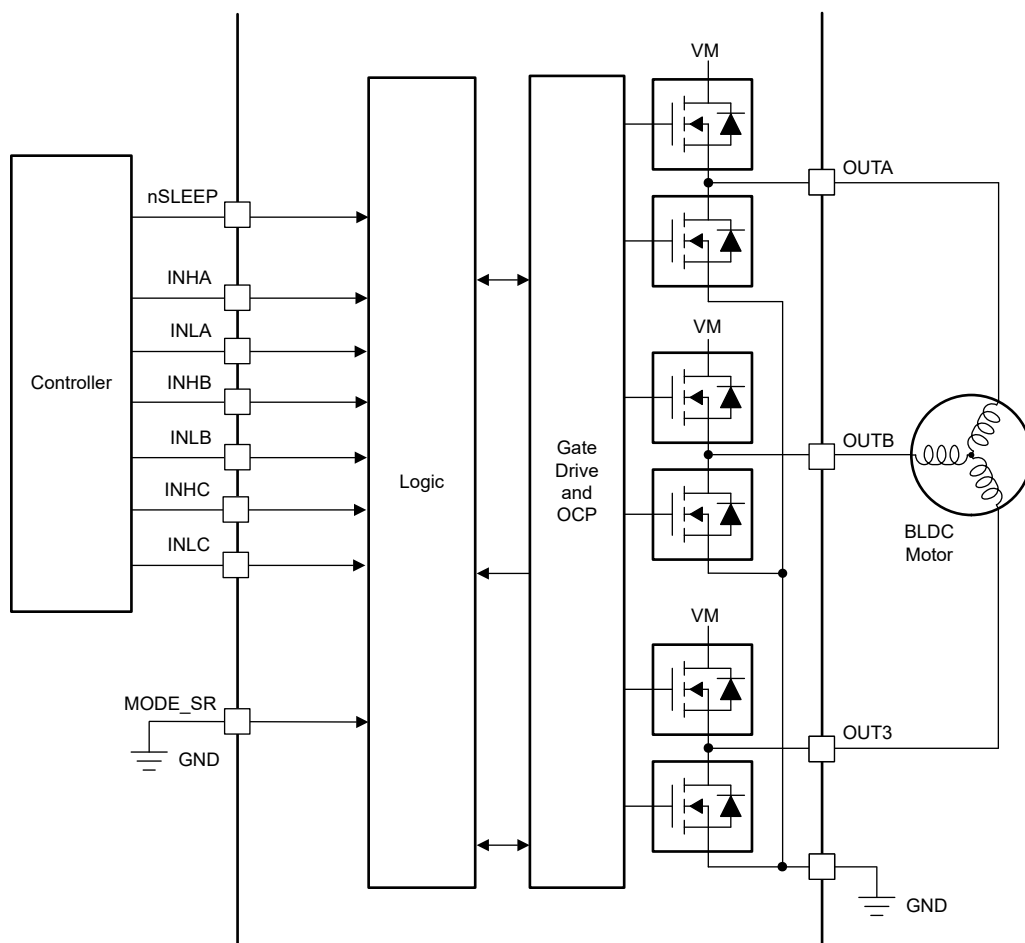
図 7-3. 6x PWM Mode
