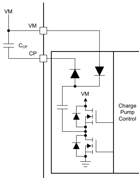
図 7-9. DRV8376 Charge Pump
