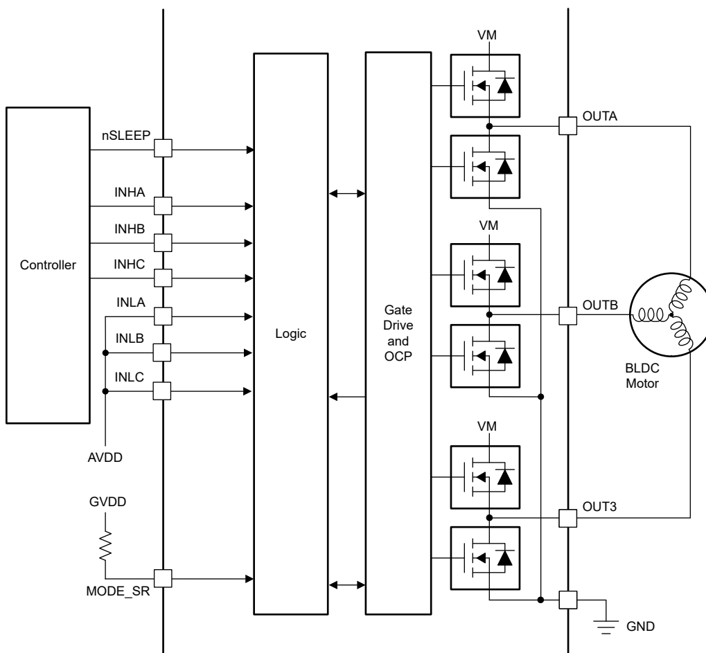
図 7-4. 3x PWM Mode
