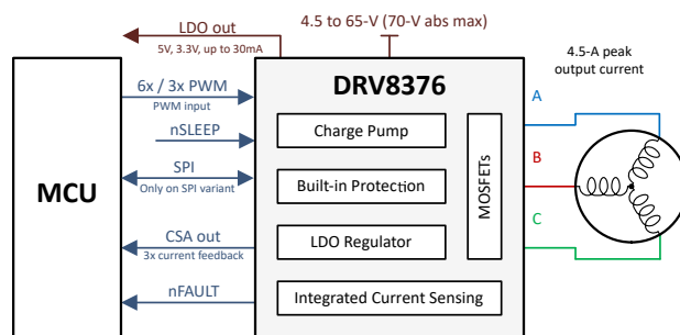
概略回路図
