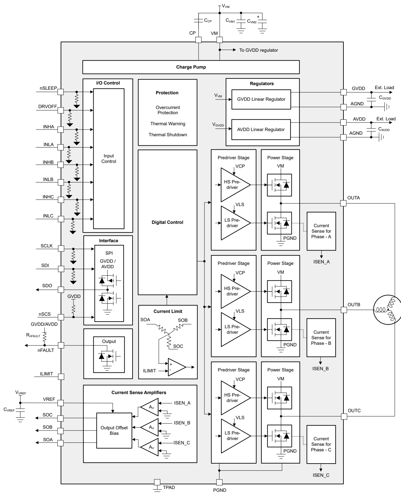
図 7-1. DRV8376S Block Diagram
