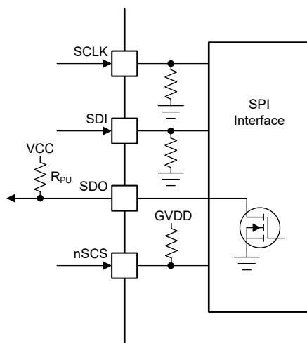
図 7-5. DRV8376S SPI Interface
