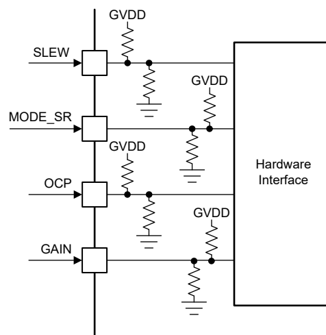
図 7-6. DRV8376H Hardware Interface
