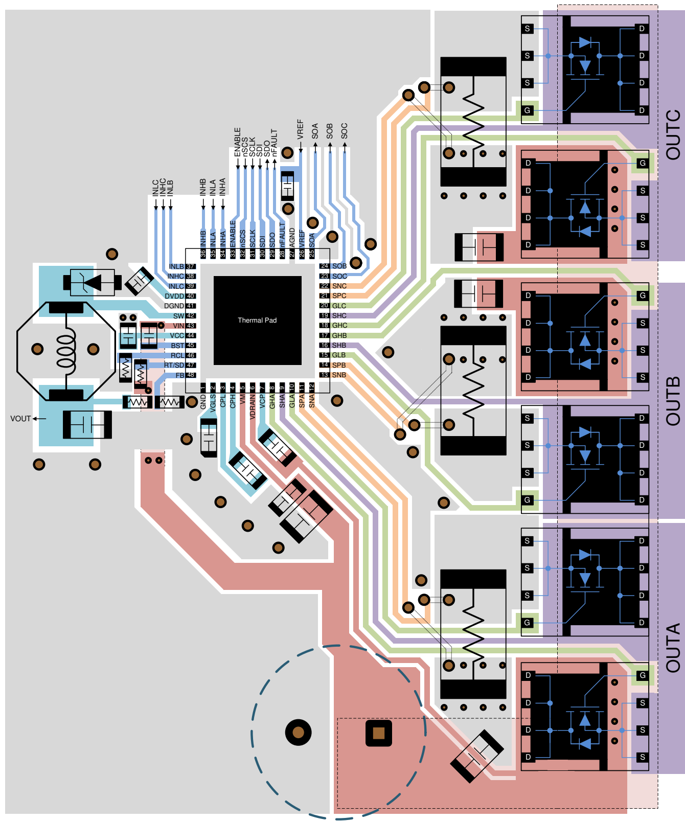
图 75. Layout Example
