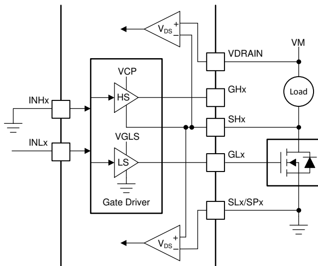
Figure 22. 1つのローサイド・ドライバ
