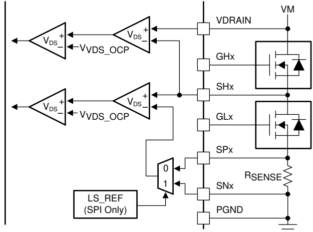
Figure 29. DRV8323とDRV8323Rの V_{DS} 監視
