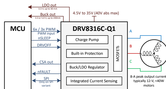
簡略回路図
