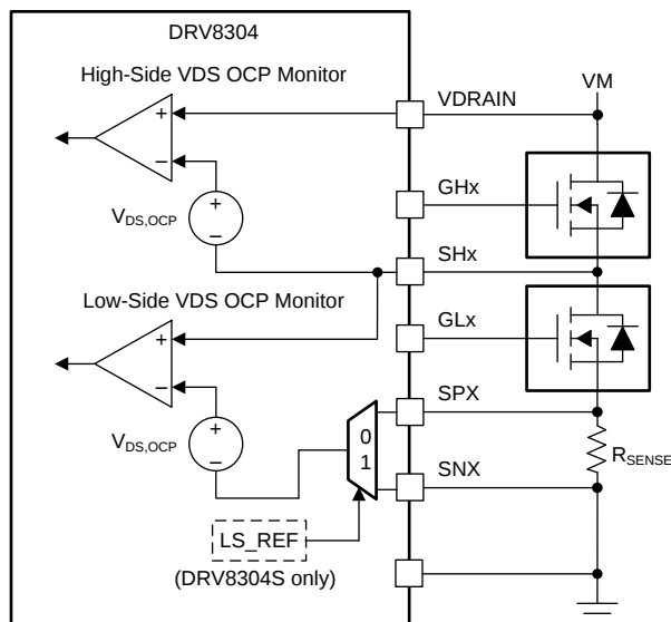
FIG 23. DRV8304 V_{DS} Monitors
