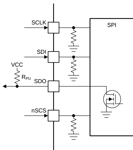
FIG 17. SPI
