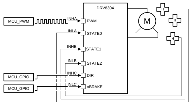
図 13. 1x PWM—Hall Sensor
