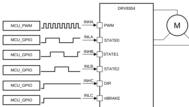
図 12. 1x PWM—Simple Controller
