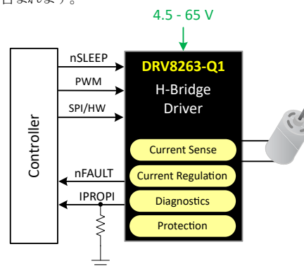
概略回路図
