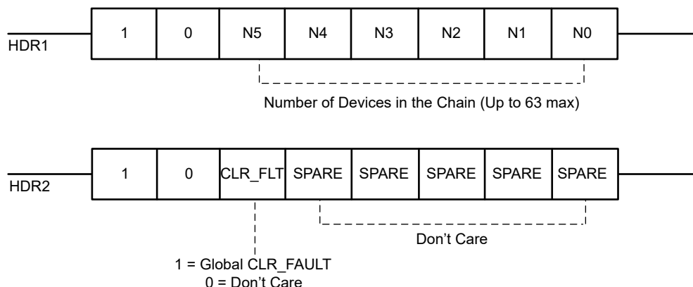
図 7-12. Header bytes
