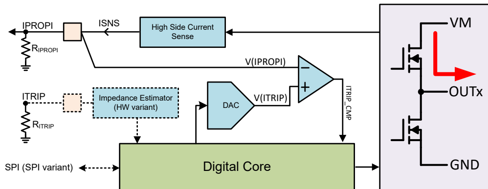
図 7-3. ITRIP Implementation
