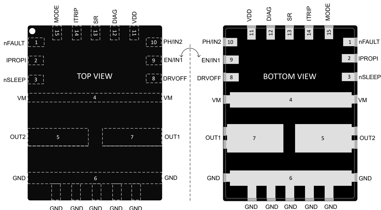
図 5-1. DRV8263H-Q1 in VQFN-HR(15) Package
