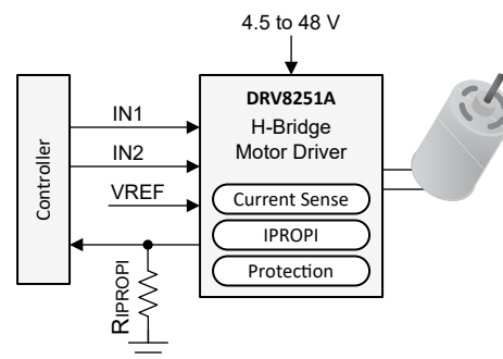
概略回路図
