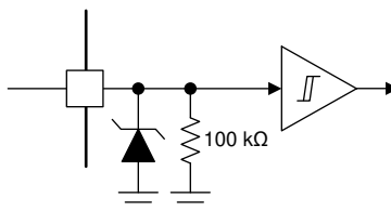
8-6. Logic-level input
