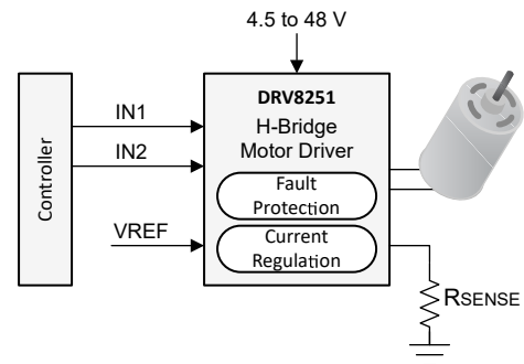
概略回路図
