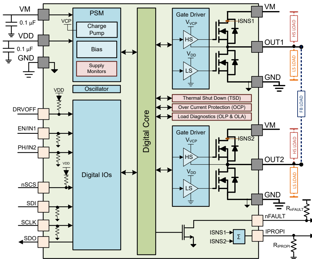
図 8-3. 機能ブロック図 - SPI (P) バリエーション
