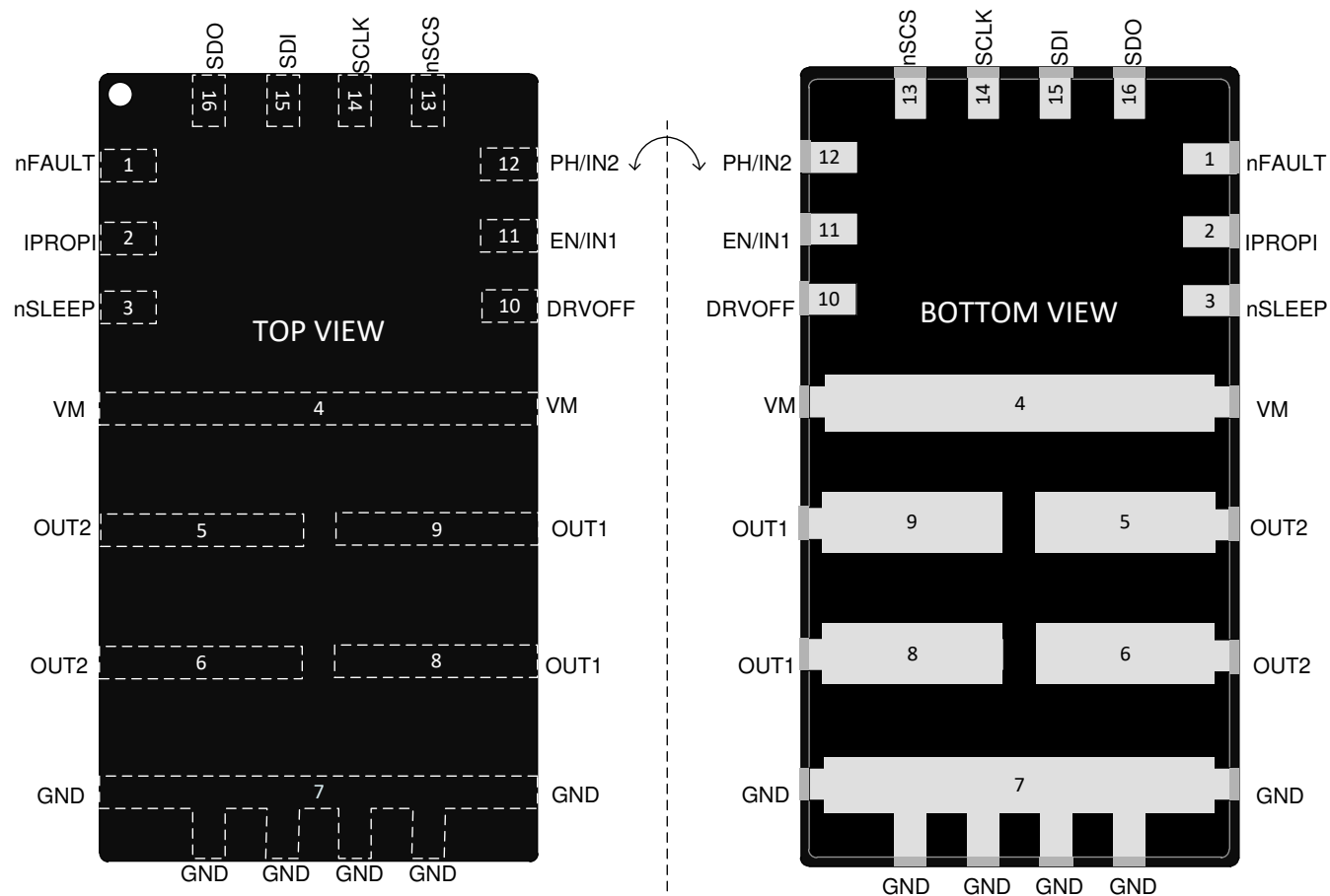
図 6-4. DRV8244S-Q1 SPI バリエーション、VQFN-HR (16) パッケージ
