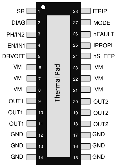
図 6-1. DRV8244H-Q1 HW バリエーション、HVSSOP (28) パッケージ
