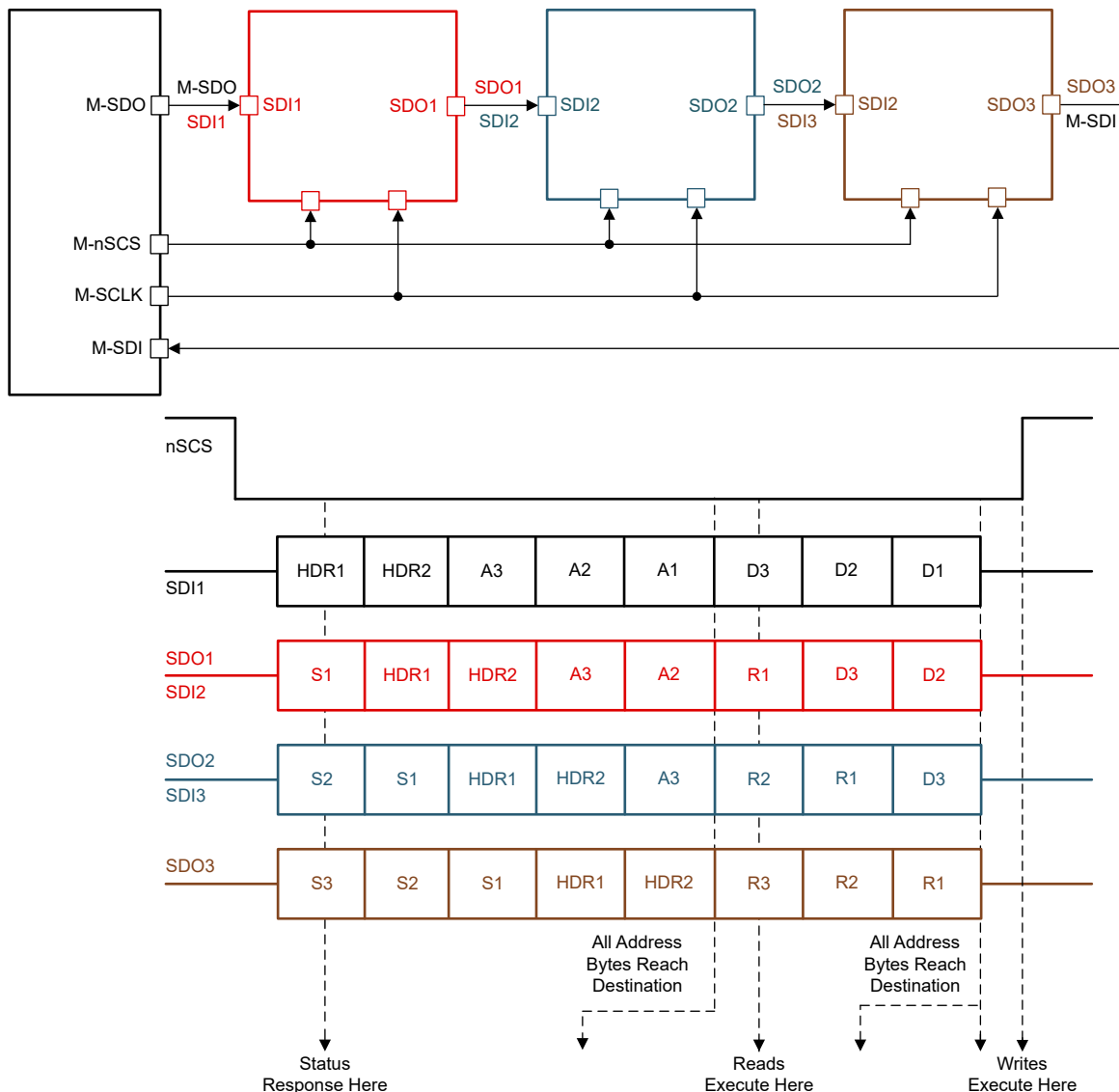
図 8-13. デジジー・チェーン SPI 動作
