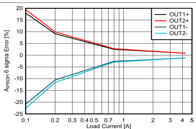
図 7-13. A_{IPROPI} ゲイン誤差と負荷電流との関係 ( V_{VM} = 13.5V )
