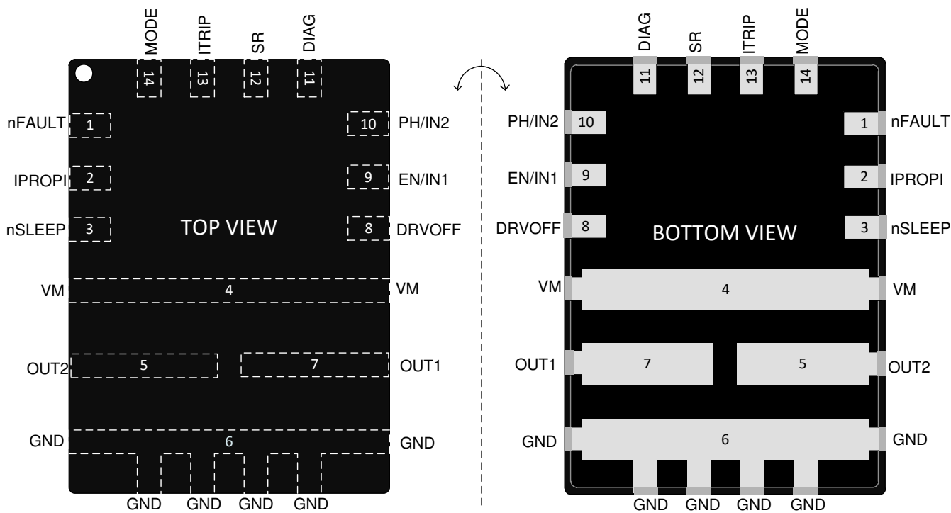
図 6-2. DRV8243H-Q1 HW バリエント、VQFN-HR (14) パッケージ
