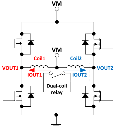
図 9-20. OUTx H ブリッジで駆動するデュアルコイル・リレーの回路図
