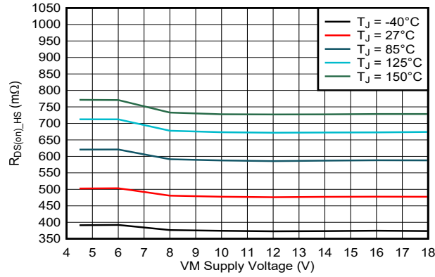
図 7-5. ハイサイド R_{DS(on)} と電源電圧との関係
