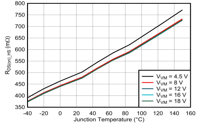
図 7-6. ハイサイド R_{DS(on)} と接合部温度 ( T_J ) との関係
