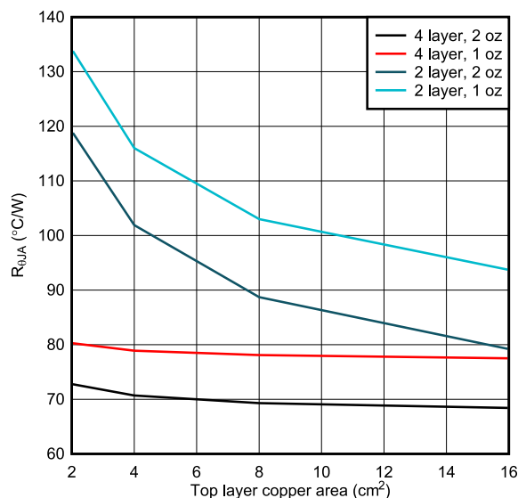
図 9-28. WSON、PCB の接合部から周囲への熱抵抗と銅面積との関係
