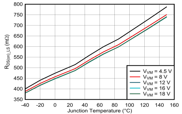
図 7-8. ローサイド R_{DS(on)} と接合部温度 ( T_J ) との関係
