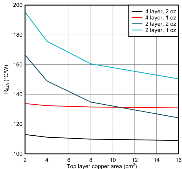
図 9-30. SOT、PCB の接合部から周囲への熱抵抗と銅面積との関係
