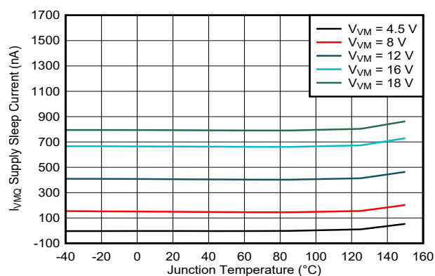
図 7-2. スリープ電流 ( I_{VMQ} ) と接合部温度 ( T_J ) との関係
