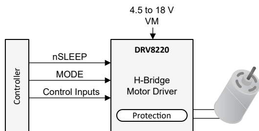
概略回路図
