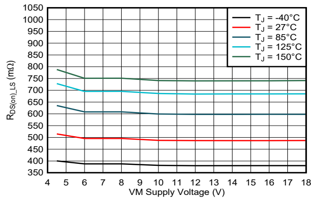
図 7-7. ローサイド R_{DS(on)} と電源電圧との関係
