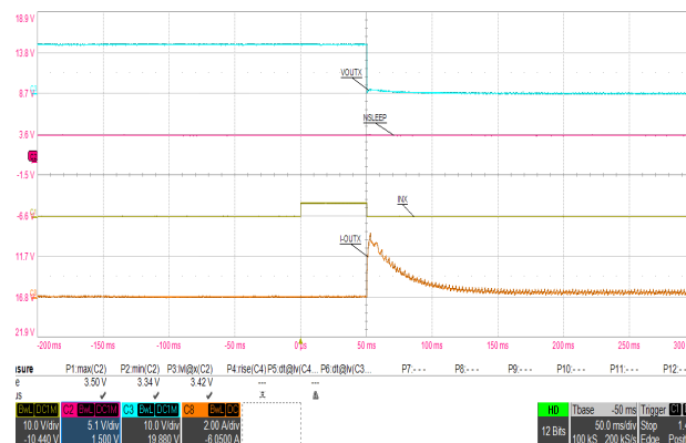
A. チャネル 1 = IN1、 IN2 (並列) チャネル 8 = モータ ー電流 チャネル 2 = V_{nSLEEP} チャネル 3 = V_{OUT} (OUT1/2 の並列)
