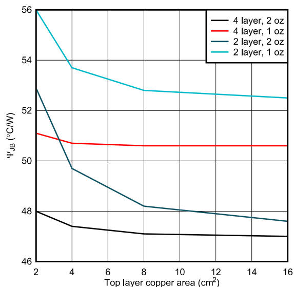
図 9-29. WSON、接合部から基板への特特性パラメータと銅面積との関係
