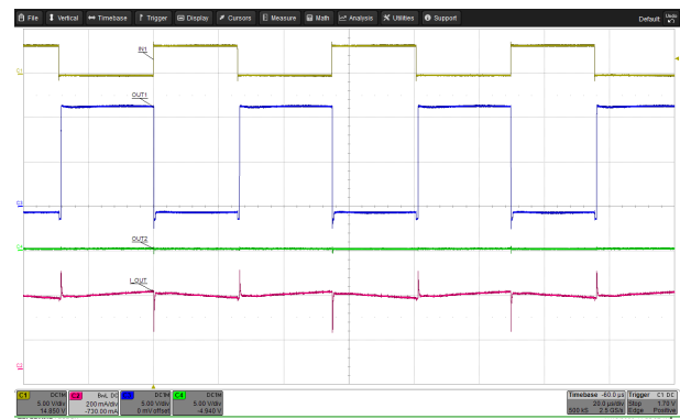
A. チャンネル 1 = IN1 チャンネル 2 = モーター電流 チャンネル 3 = OUT1 チャンネル 4 = OUT2
