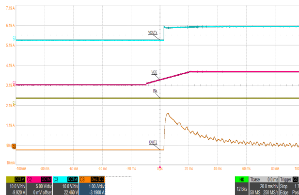
A. チャンネル 1 = IN1、チャンネル 2 = V VCC チャンネル 3 = V OUT (OUT1/2 の並列) チャンネル 8 = モーター 一電流
