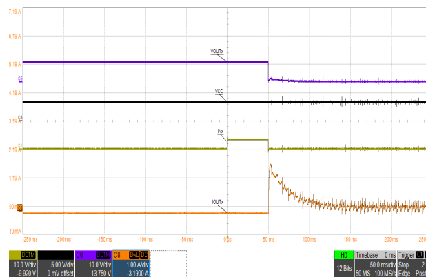
A. チャンネル 1 = IN1、チャンネル 5 = V VCC チャンネル 6 = V OUT (OUT1/2 の並列) チャンネル 8 = モーター 一電流
