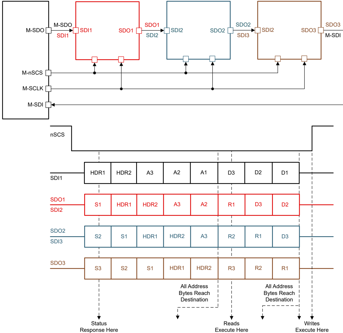
図 7-10. デジィー・チェーン SPI 動作
