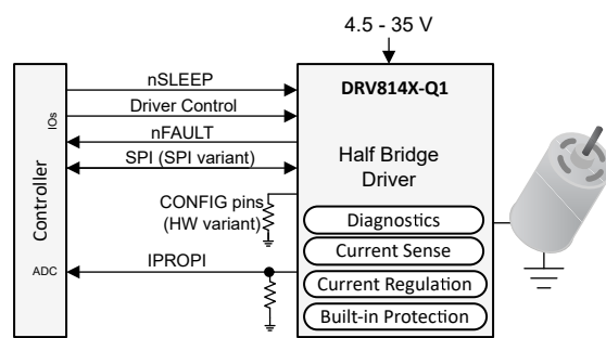
概略回路図
