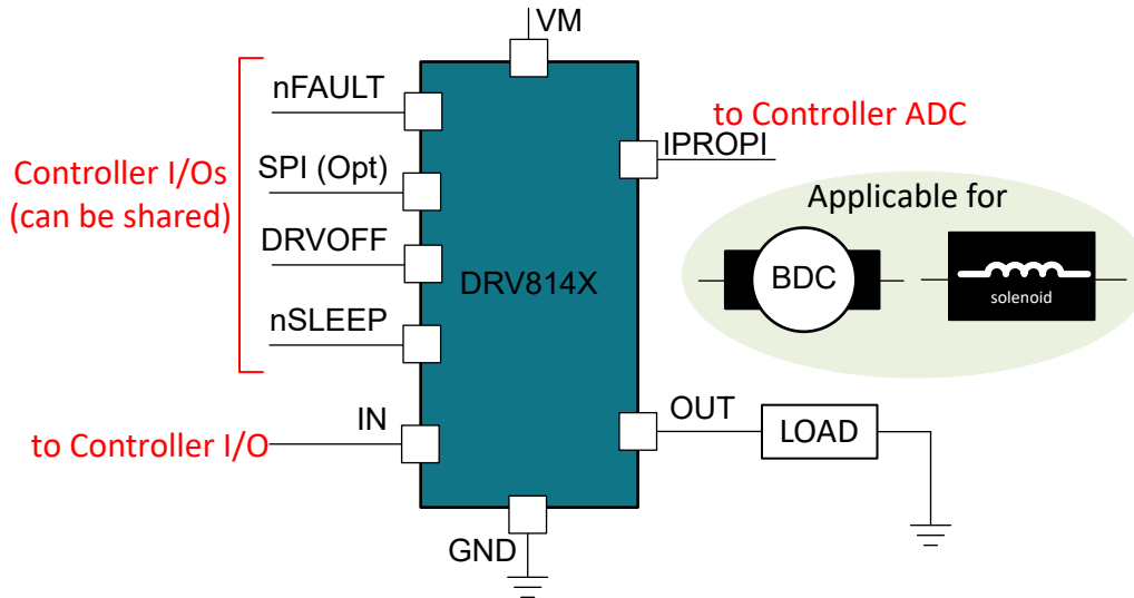
図 9-2. DRV8144x-Q1 デバイスでローサイド負荷を駆動するハーフブリッジ・トポロジの説明図
