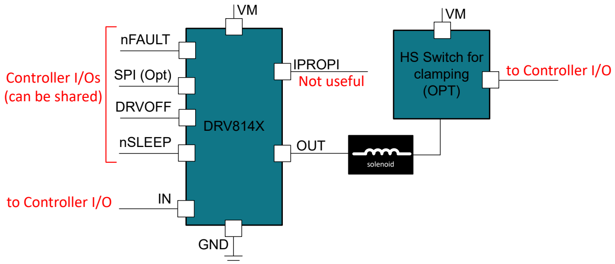
図 9-3. DRV8144x-Q1 デバイスでハイサイド負荷を駆動するハーフブリッジ・トポロジの説明図
