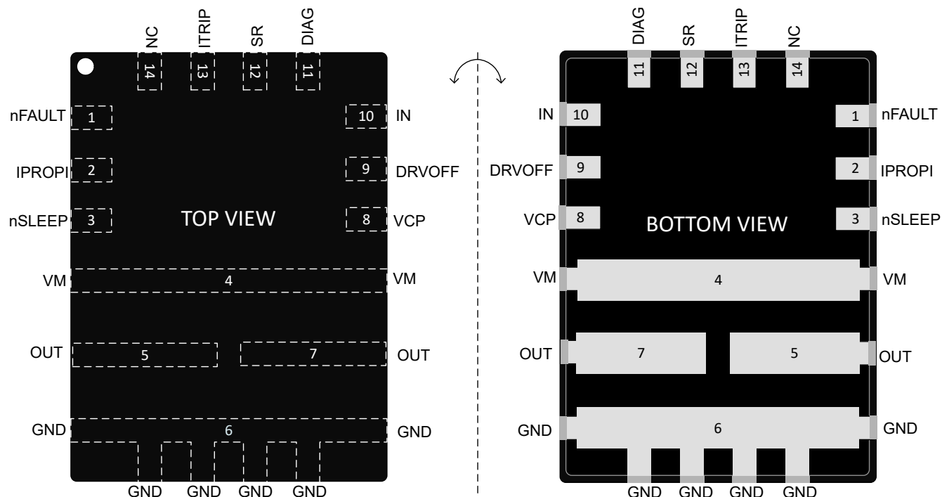
図 5-1. DRV8143H-Q1 HW バリエント、VQFN-HR (14) パッケージ
