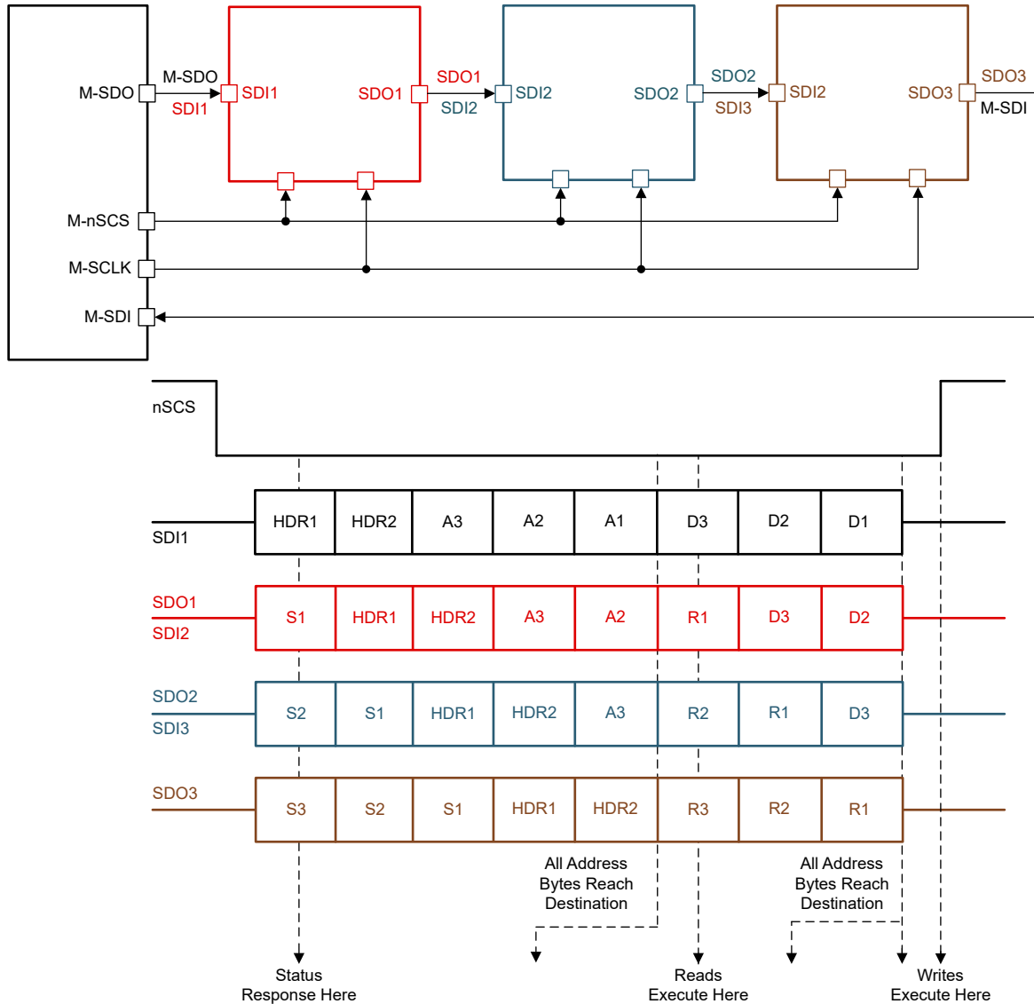
図 7-11. デジジー・チェーン SPI 動作
