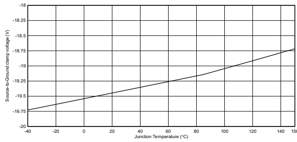
図 6-6. ソース-グランド間クランプ電圧
