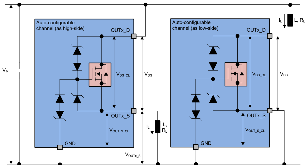
図 7-9. 自動構成可能チャネルの出力クランプ
