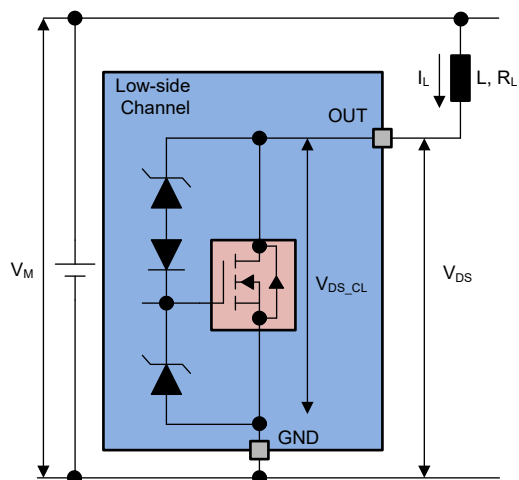
図 7-8. ローサイド チャネルの出力クランプ
