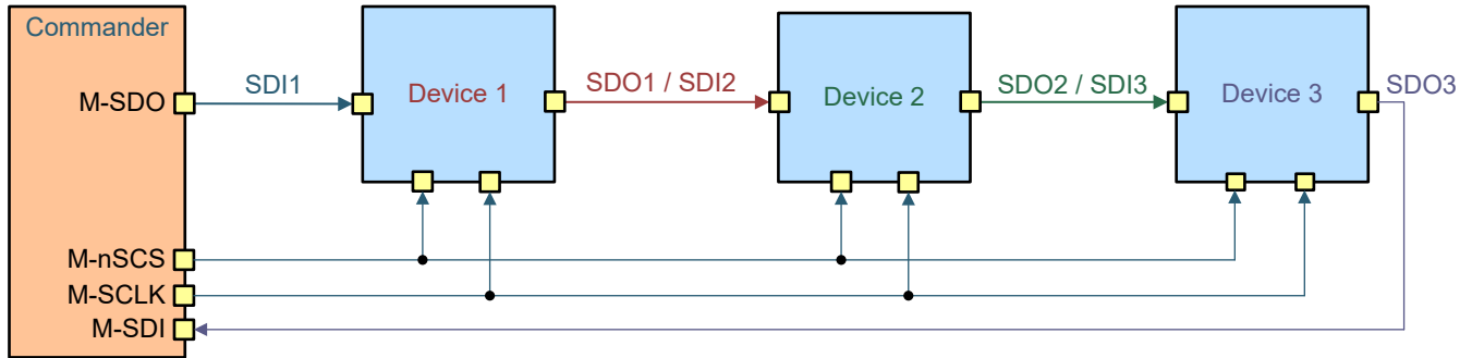
図 7-26. デイジー チェーン構成
