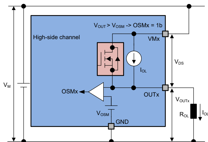
図 7-21. 出力ステータス モニタ - ハイサイド チャネル
