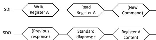
図 7-28. レジスタの内容をマイクロコントローラに送り返します
