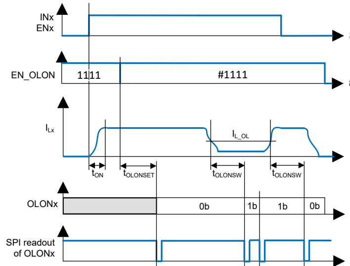
図 7-22. オン時の開放負荷 (直接チャネル診断)
