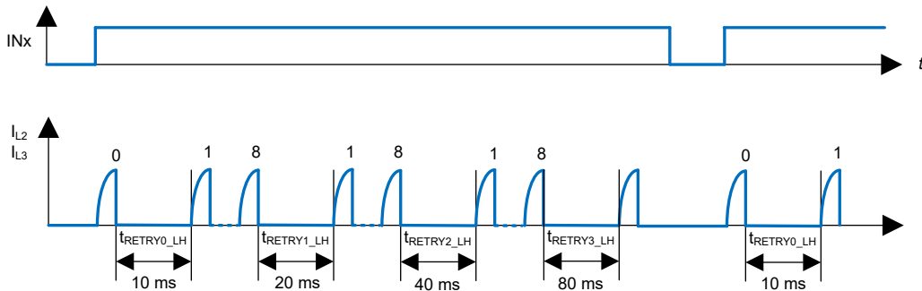
図 7-16. リンプホームでタイマーを再起動します
