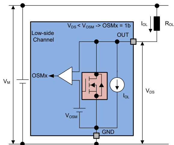
図 7-18. 出力ステータス モニタ - ローサイド チャンネル
