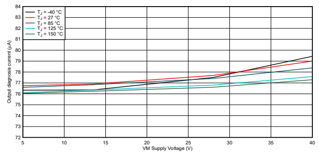
図 6-9. 出力診断電流、 V_{DD} = 5.5\text{ V}
