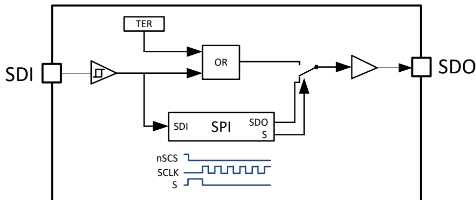
図 7-25. TER ビットの組み合わせロジック
