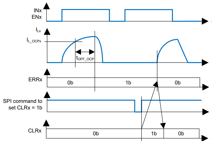
図 7-15. 過電流時にラッチオフする
