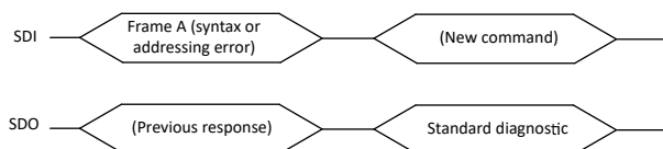
図 7-31. コマンド構文エラー後の応答
