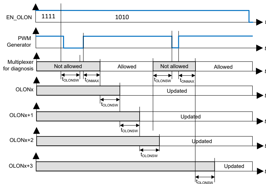
図 7-24. オン時開放負荷診断のタイミング (診断ループ - 内部 PWM ジェネレータ制御チャネル)
