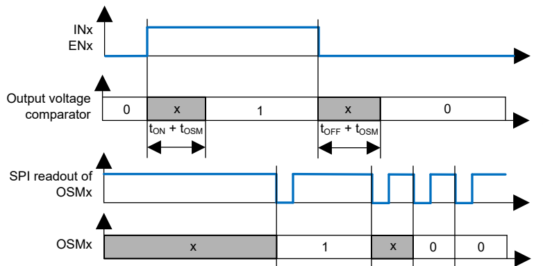
図 7-17. 出力ステータス モニタ タイミング
