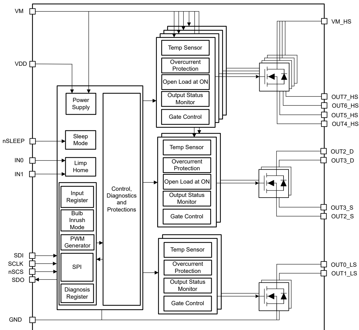
図 7-1. DRV81242-Q1 の機能ブロック図
