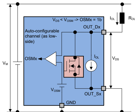
図 7-20. 出力状態モニタ - ローサイド構成時自動構成可能チャネル
