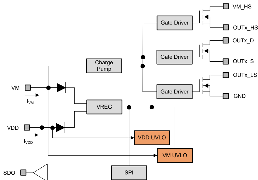
図 7-3. 内部電源アーキテクチャ
