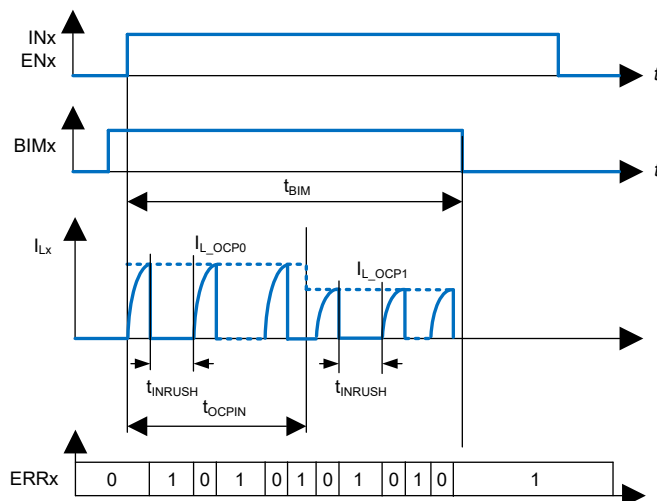
図 7-11. 電球突入モード (BIM) 動作
