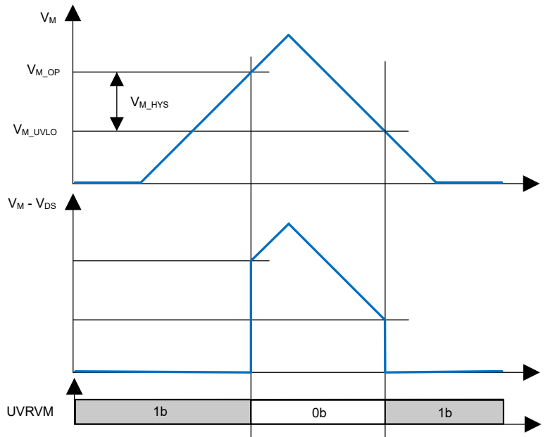
図 7-13. V_M 低電圧の動作
