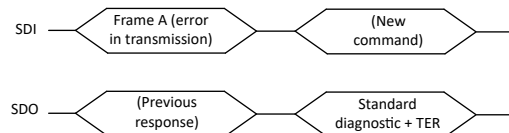
図 7-29. 送信エラー後の応答
