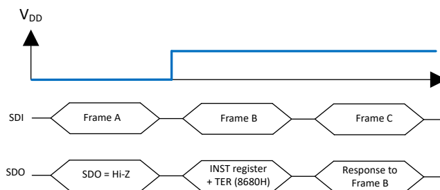
図 7-30. V DD でのパワーオン リセットから復帰した後の応答
