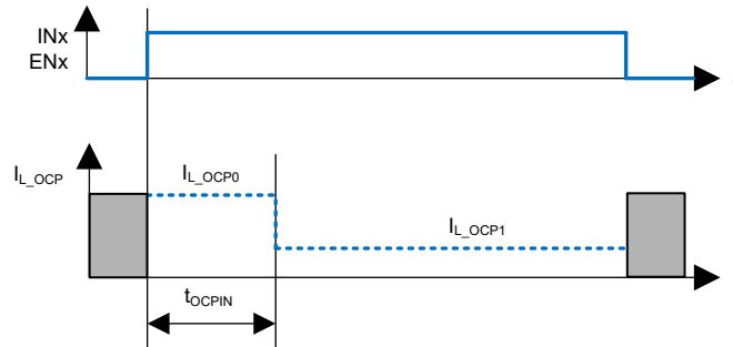
図 7-14. 過電流スレッシュホールド
