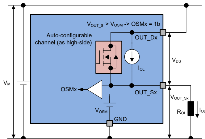
図 7-19. 出力ステータスマニタ - ハイサイド構成時自動構成可能チャネル
