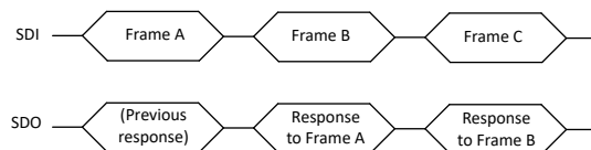
図 7-27. SPI 通信中の SDI と SDO の関係
