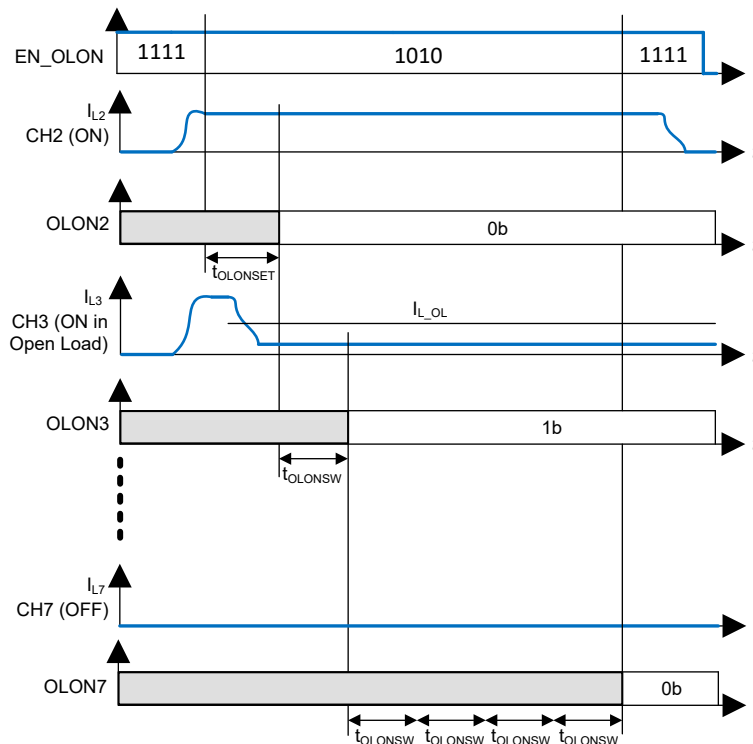
図 7-23. オン時間開放負荷診断のタイミング (診断ループ - マイコン制御チャンネル)
