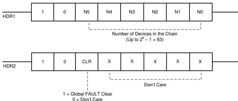
図 7-22. ヘッダ・ビット
