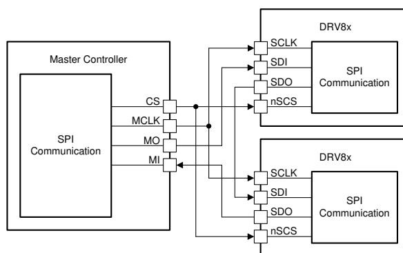
図 7-20. デジジー・チェーンを使った SPI 動作
