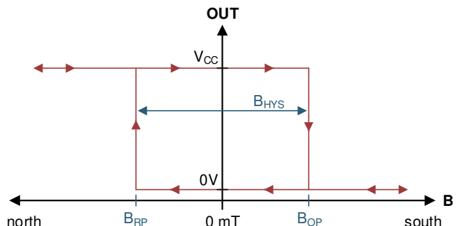
磁気応答
