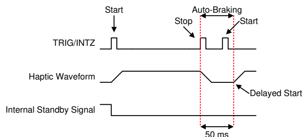
図 7-23. トリガ パルスと遅延スタート (RTP または波形シーケンサ)
