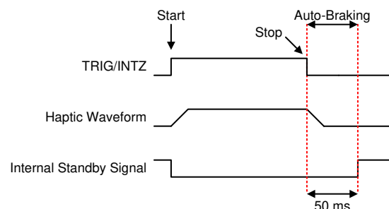
図 7-20. 再生開始および停止トリガ (レベル) (RTP または波形シーケンサ)
