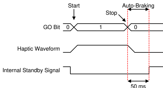
図 7-21. 再生の開始および停止トリガ (内部 GO ビット) (RTP または波形シーケンサ)
