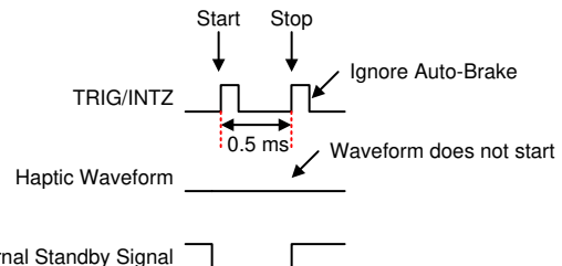
図 7-18. トリガ パルス (RTP または波形シーケンサ) による高速スタート ストップ
