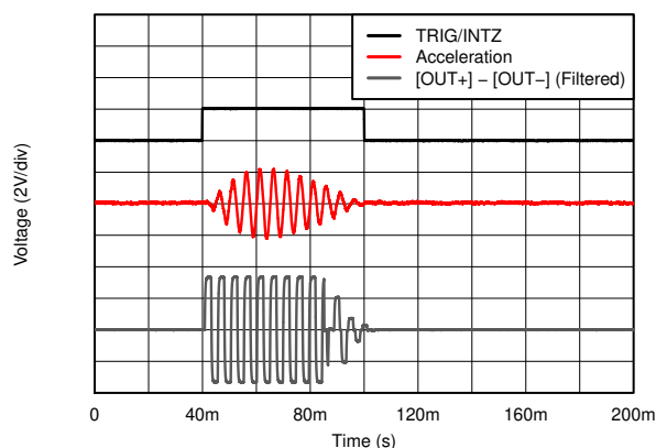
図 5-9. ERM RTP バズ (クローズドループ)、パルストリガ付き
