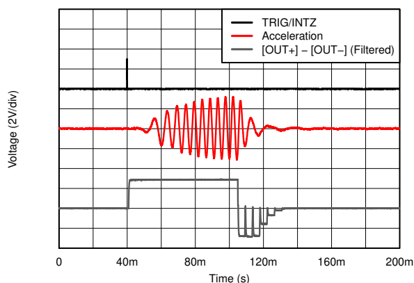
図 5-10. LRA 正弦波クリック (開ループ) と自動ブレーキ
