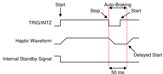
図 7-22. 遅延スタート付きトリガ レベル (RTP または波形シーケンサ)
