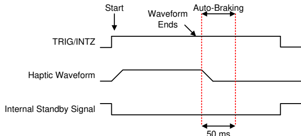
図 7-17. TRIG/INTZ ピンが high のままになったときのトリガ レベル動作を備えた波形シーケンサ
