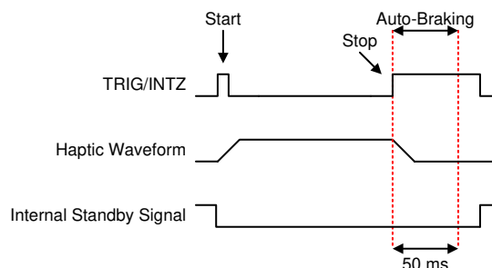
図 7-26. TRIG/INTZ ピンが high のままのとき (RTP または波形シーケンサ)、トリガ パルス動作
