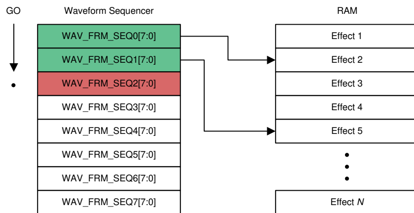
図 7-14. 波形シーケンサのプログラミング
