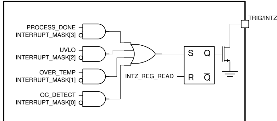
図 7-6. 割り込みモードの TRIG/INTZ 機能
