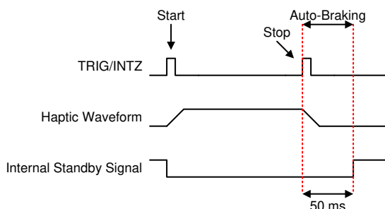
図 7-19. 再生開始および停止トリガ (パルス) (RTP または波形シーケンサ)
