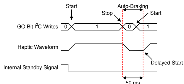
図 7-25. 遅延スタート付き GO ビット トリガ (RTP または波形シーケンサ)
