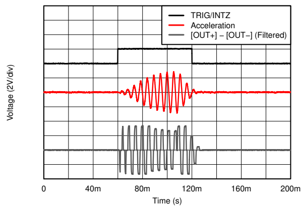
図 5-4. ERM と LRA の起動レイテンシ
