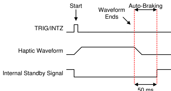
図 7-15. トリガ パルス付き波形シーケンサ
