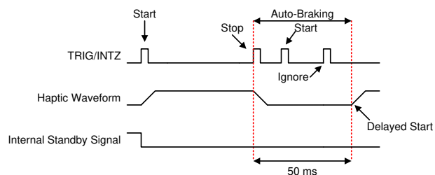
図 7-24. トリガ パルスと遅延スタート、無視されたパルス (RTP または波形シーケンサ)
