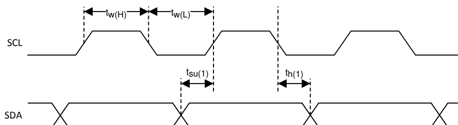
図 5-1. SCL と SDA のタイミング
