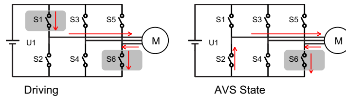
FIG 37. Inductive AVS
