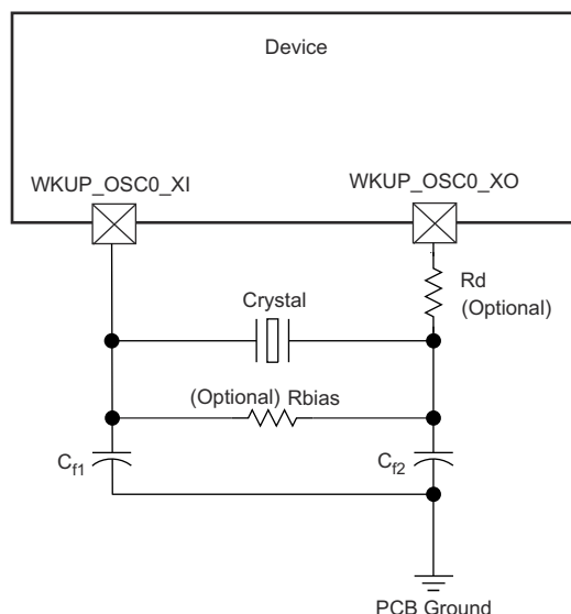
図 6-23. WKUP_OSC0 Crystal Implementation
