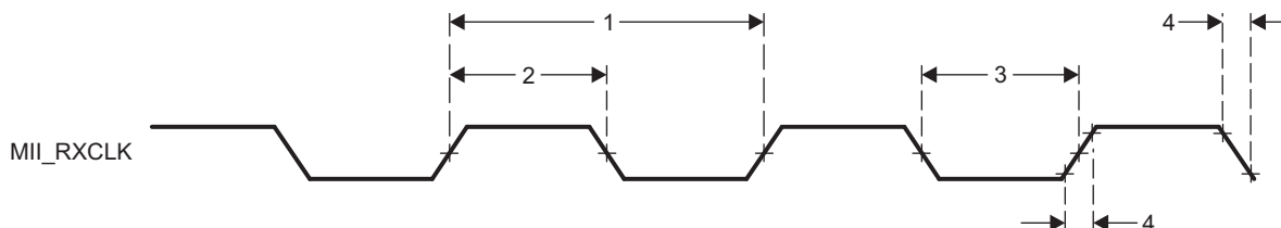
图 5-125. PRU-ICSS MII[x]_RXCLK Timing
