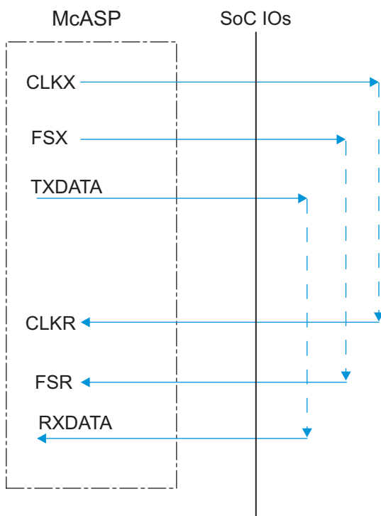
FIG 5-59. McASP1-8 COIFOI – ASYNC Mode
