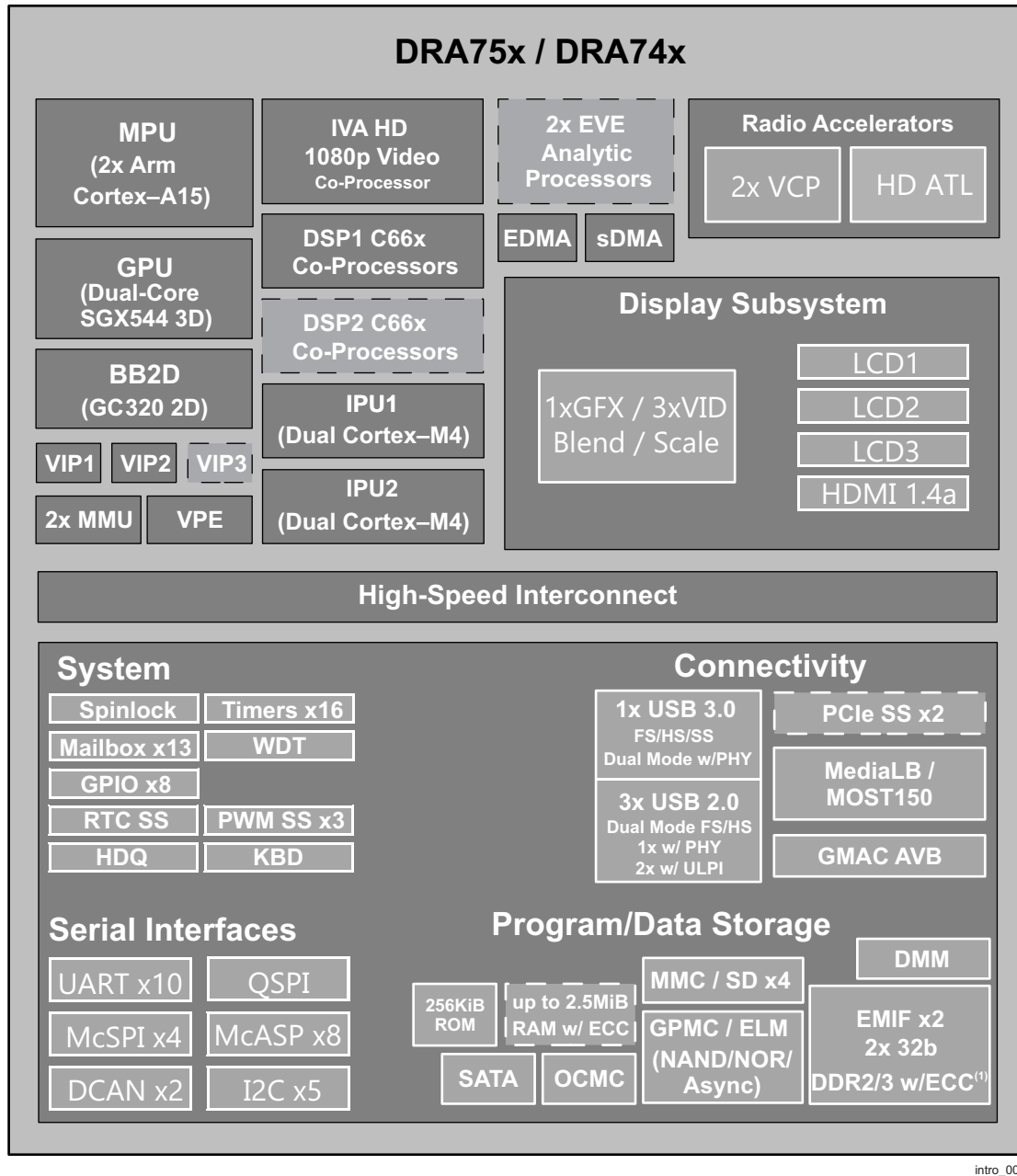
図 1-1. DRA75x、DRA74xのブロック図
