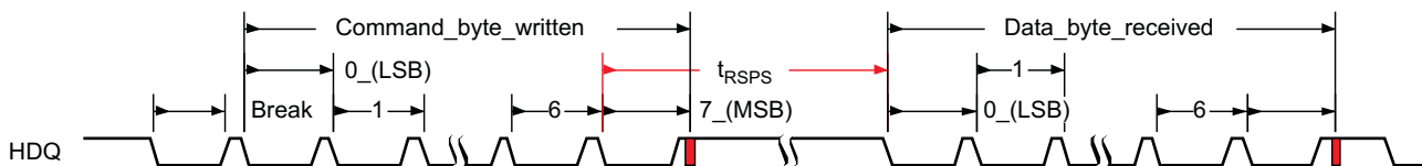
图 7-28. HDQ Communication Timing
