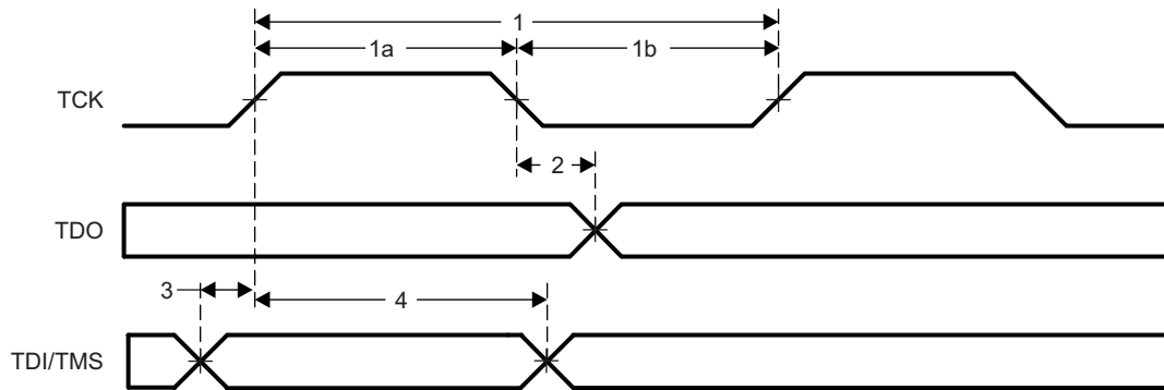
图 7-94. JTAG Timing
