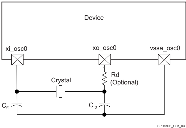
6-2. OSC0 Crystal Implementation
