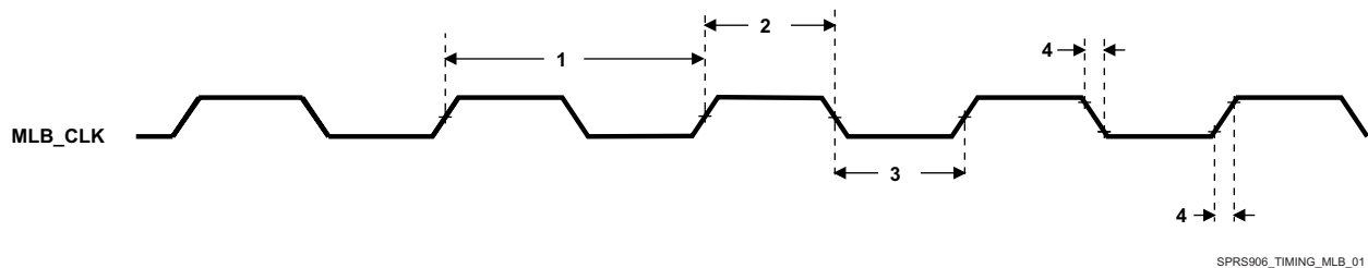
图 7-61. MLB_CLK Timing
