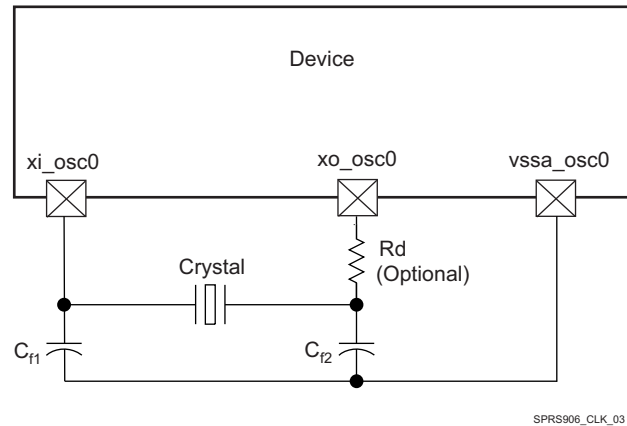
6-2. OSC0 Crystal Implementation
