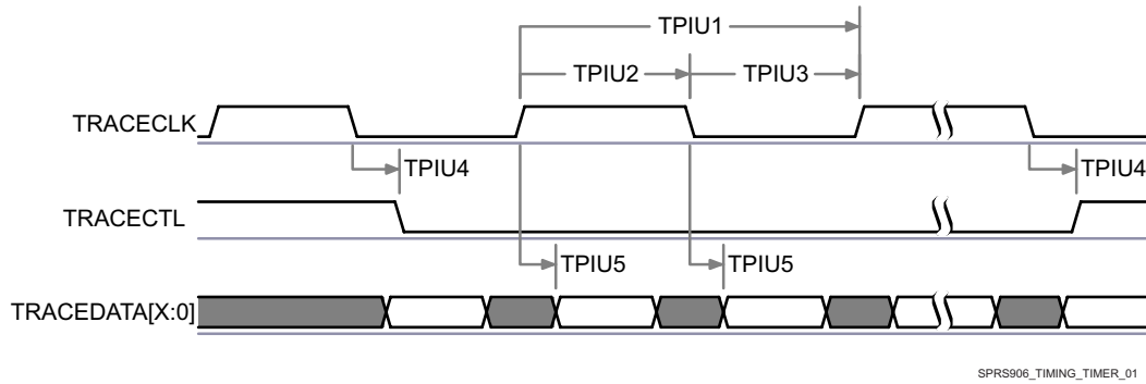
图 7-96. TPIU-PLL DDR Transmit Mode (1)
