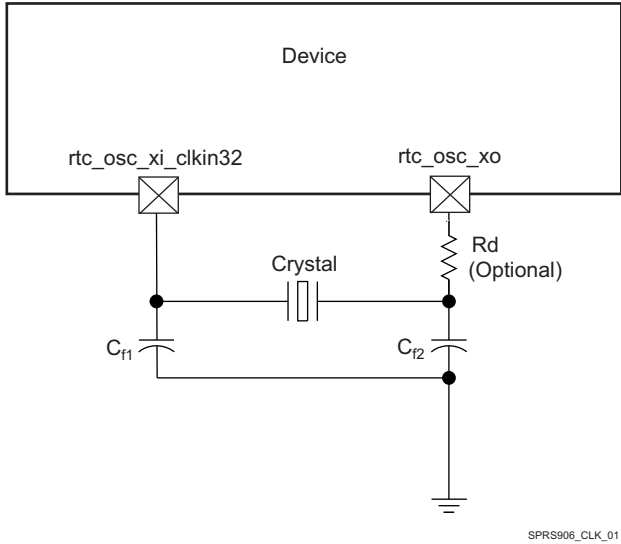
图 6-10. Crystal Implementation
