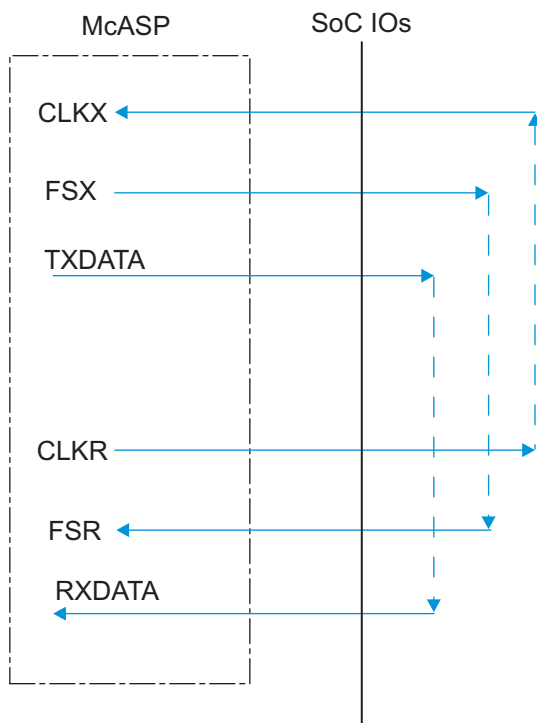
FIG 5-62. McASP1-8 CIOFOI – ASYNC Mode
