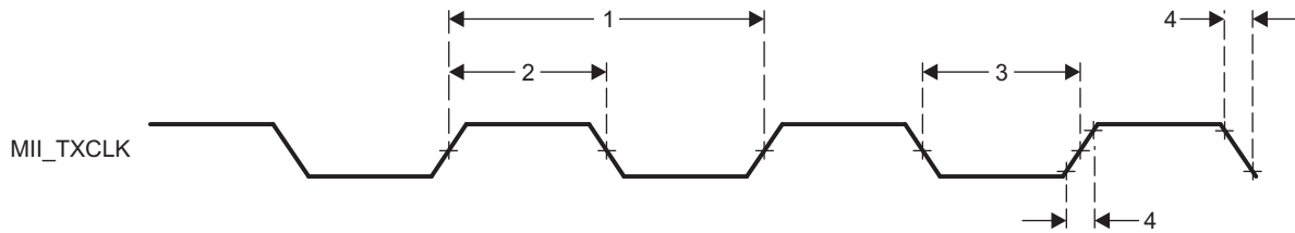
图 5-126. PRU-ICSS MII[x]_TXCLK Timing
