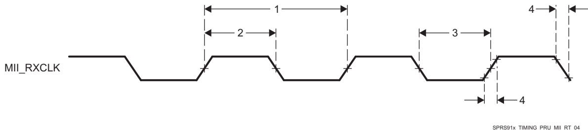
图 5-125. PRU-ICSS MII[x]_RXCLK Timing
