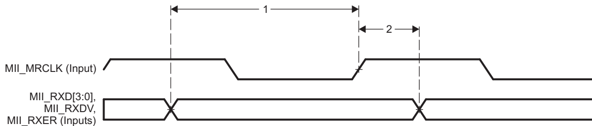
图 5-127. PRU-ICSS MII_RXD[3:0], MII_RXDV, and MII_RXER Timing
