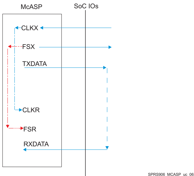
图 5-64. McASP1-8 CI-FO- – SYNC Mode
