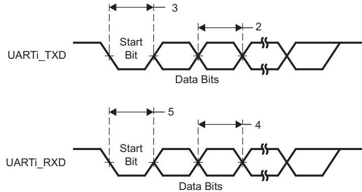
図 5-48. UART Timing
