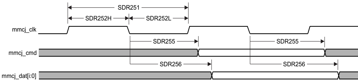
图 5-106. MMC/SD/SDIOj in - SDR25 - Transmitter Mode
