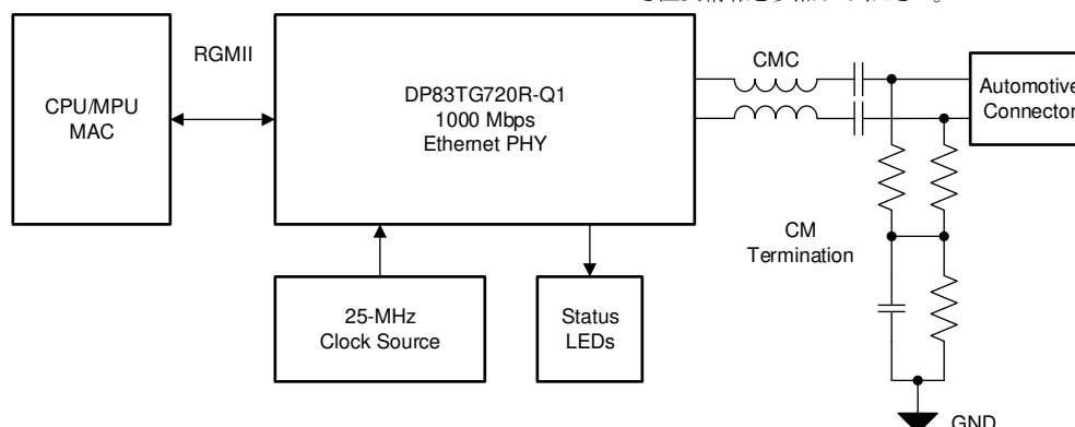
図 3-1. 概略回路図
