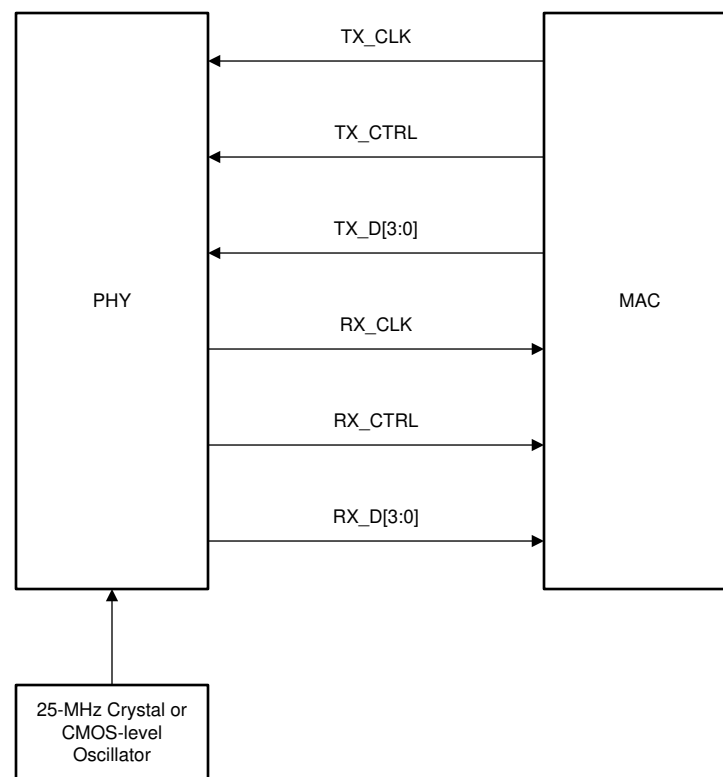
図 8-13. RGMII の接続
