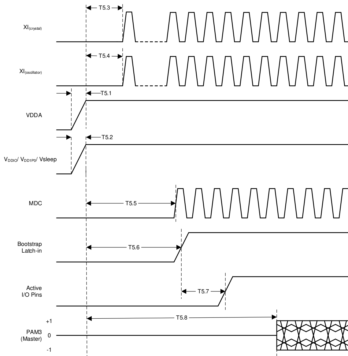
図 7-1. 電源投入タイミング
