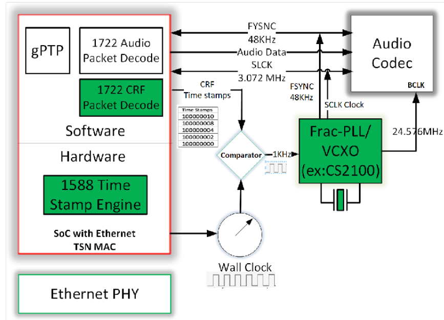
図 5-5. 代表的なオーディオ オーバー イーサネット アーキテクチャ
