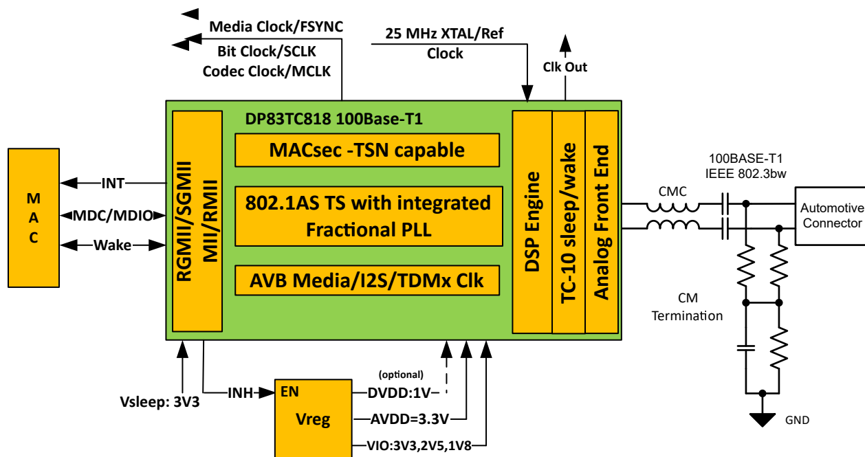
概略回路図
