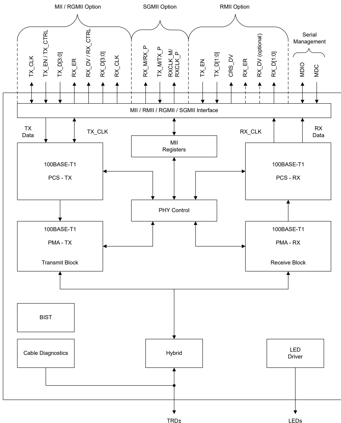
图 8-1. DP83TC814S-Q1
