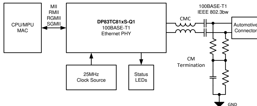
概略回路図
