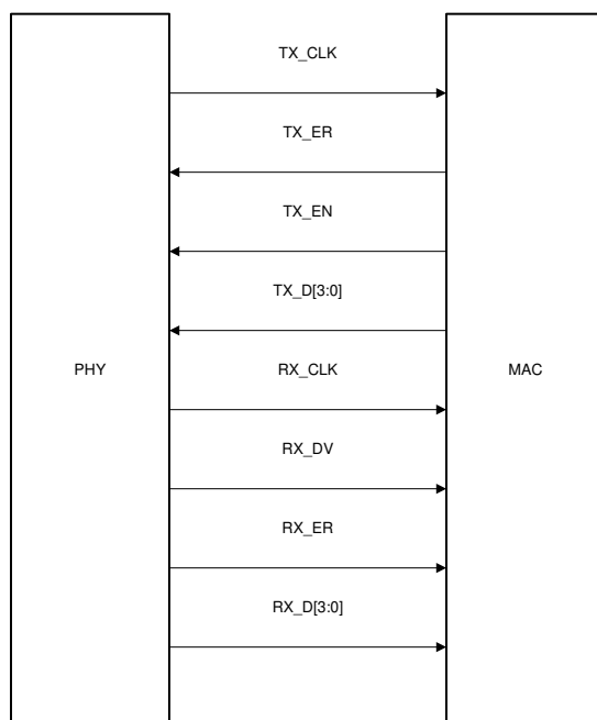
图 8-11. MII Signaling
