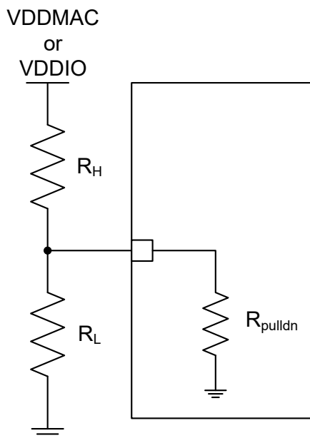
图 8-14. Strap Circuit
