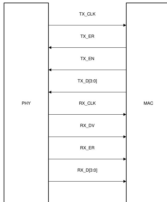
图 8-14. MII Signaling
