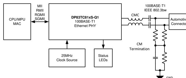
概略回路図
