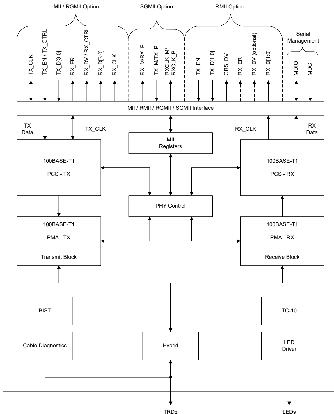
図 7-1. DP83TC812S-Q1
