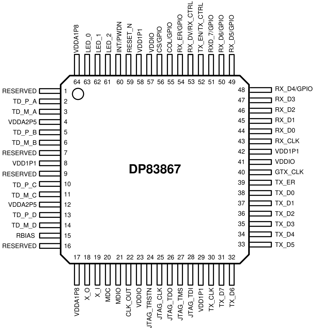
図 5-1. PAP Package
