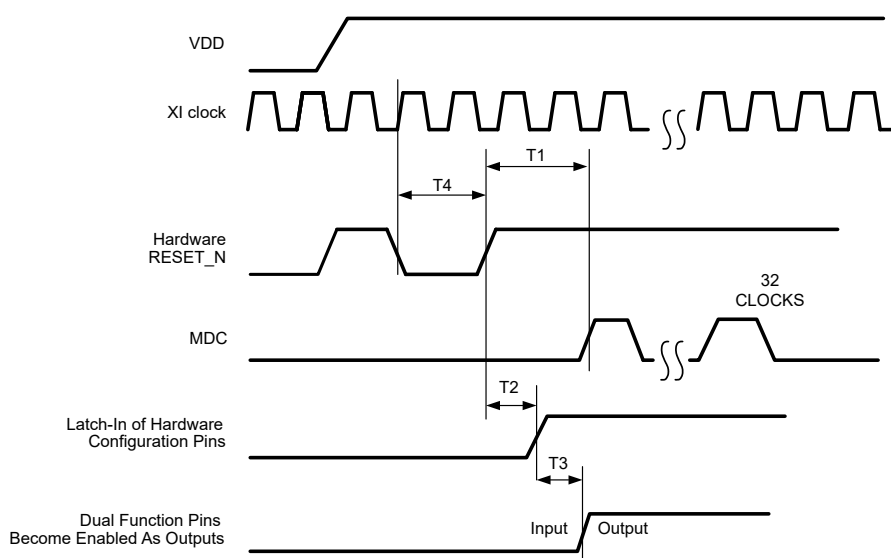
图 6-2. Reset Timing
