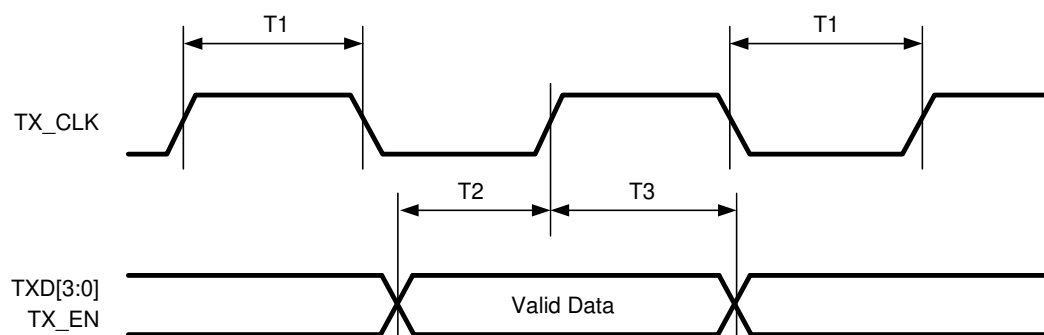
図 6-8. 100Mbps MII Transmit Timing
