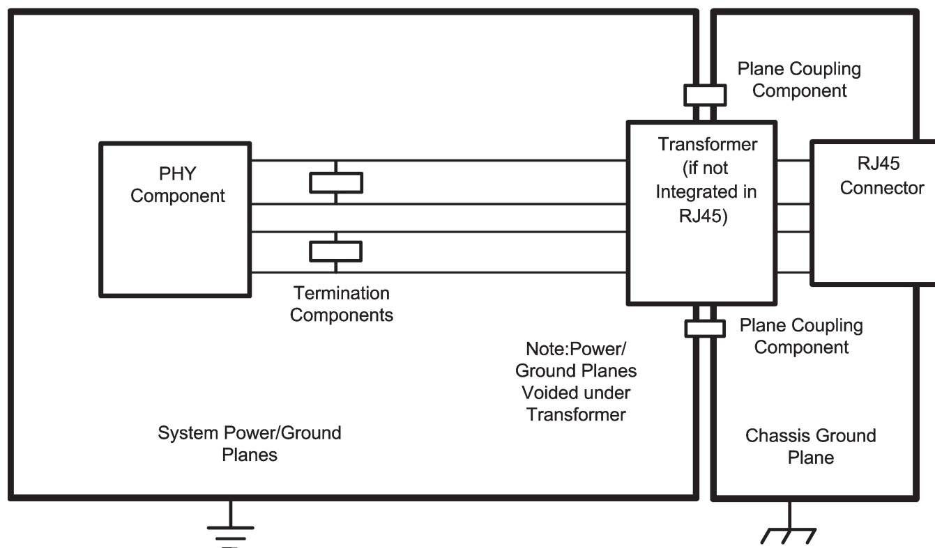
图 8-5. Layout Example
