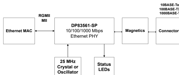
標準的なイーサネット・システムのブロック図
