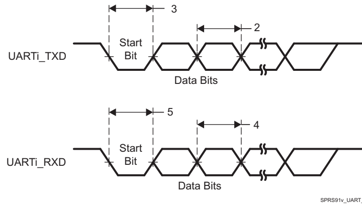
図 5-40. UART Timing
