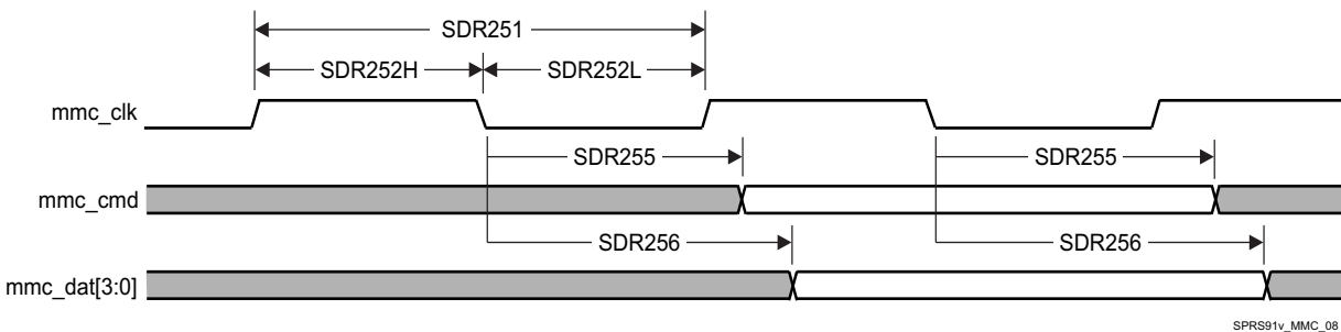
図 5-61. MMC/SD/SDIOj in - SDR25 - Transmitter Mode
