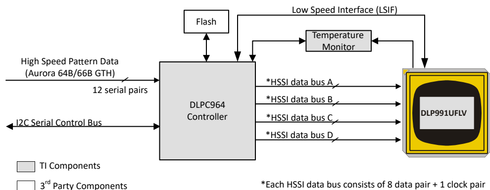
アプリケーション概略図
