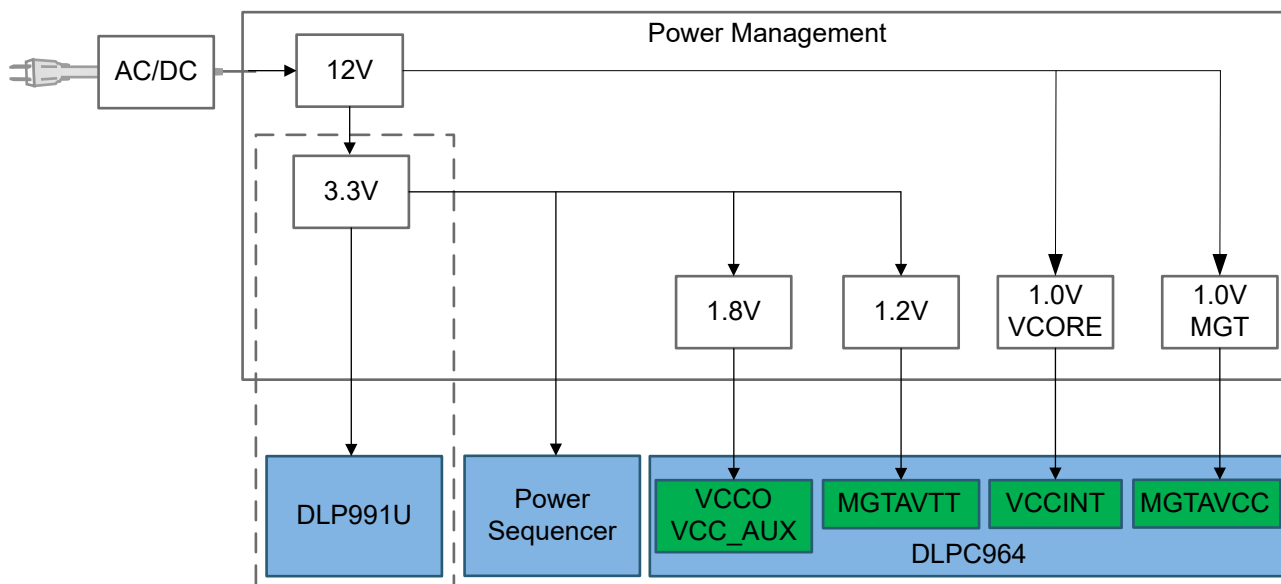
図 7-11. Power Distribution
