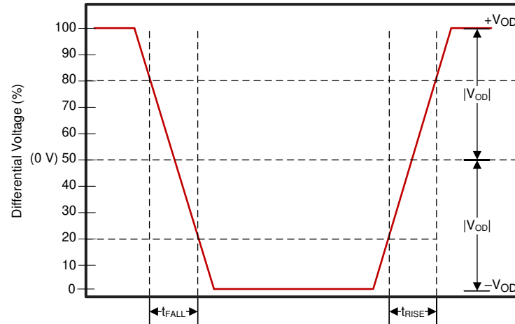
図 6-3. 差動出力信号
