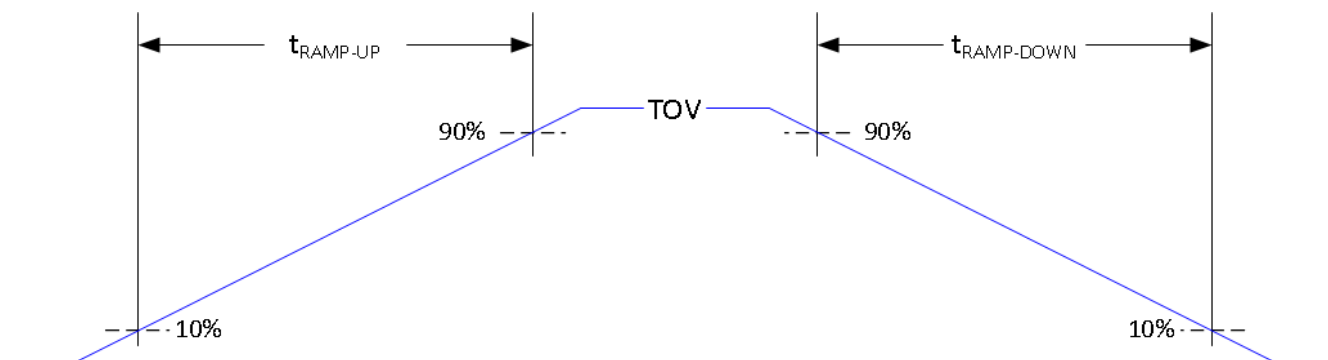
図 6-7. 電源ランプ時間
