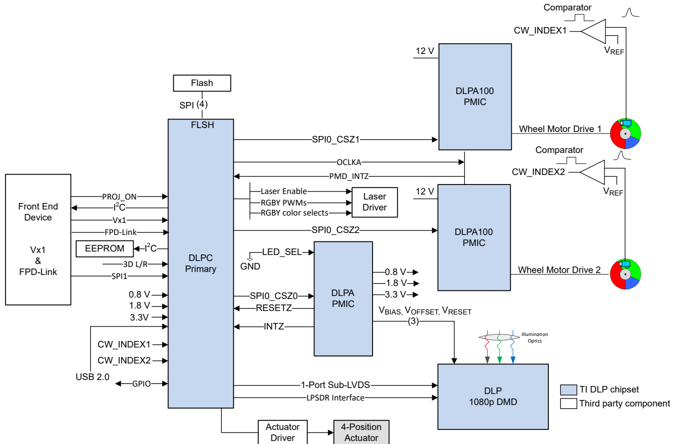
図 7-2. レーザー蛍光の機能ブロック図
