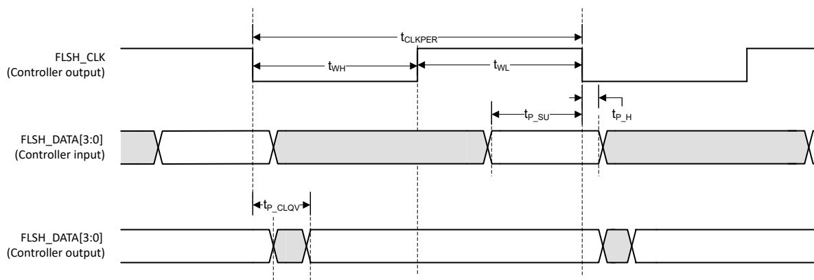
図 6-9. フラッシュ インターフェイスのタイミング
