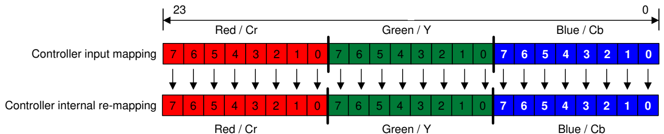
図 6-2. RGB-888 I/O Mapping
