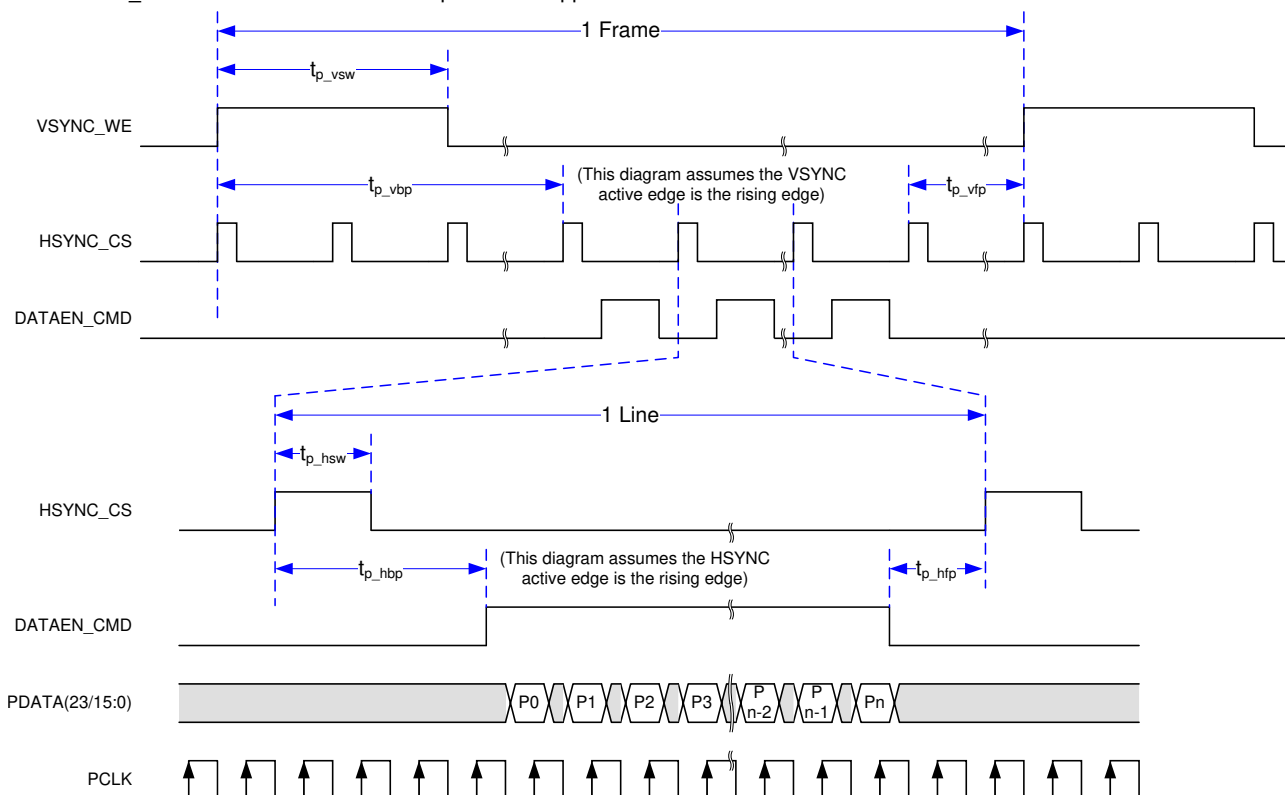
図 5-7. Parallel Interface Frame Timing
