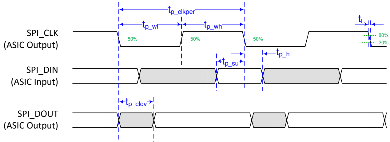
5-9. TPS99000-Q1 Interface Timing
