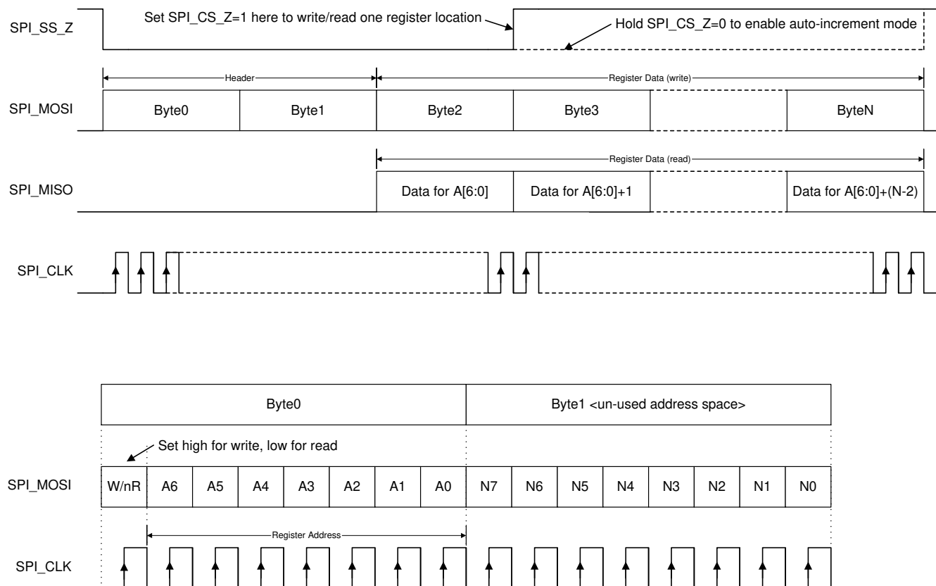
図 6-10. SPI Protocol
