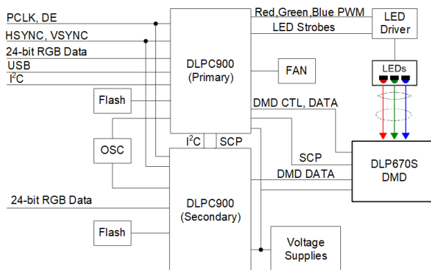
DLP670S の概略回路図
