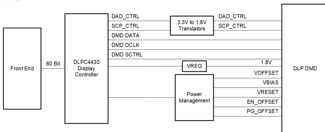
DLP650NE のアプリケーション概略図
