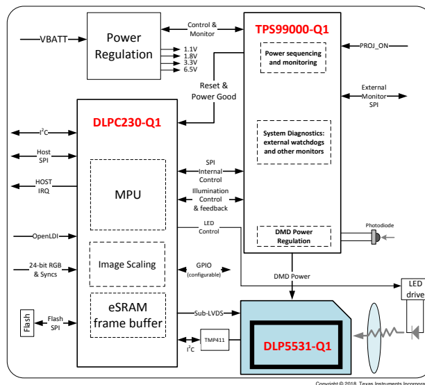
DLP5531-Q1 DLP®チップセットのシステム・ブロック図
