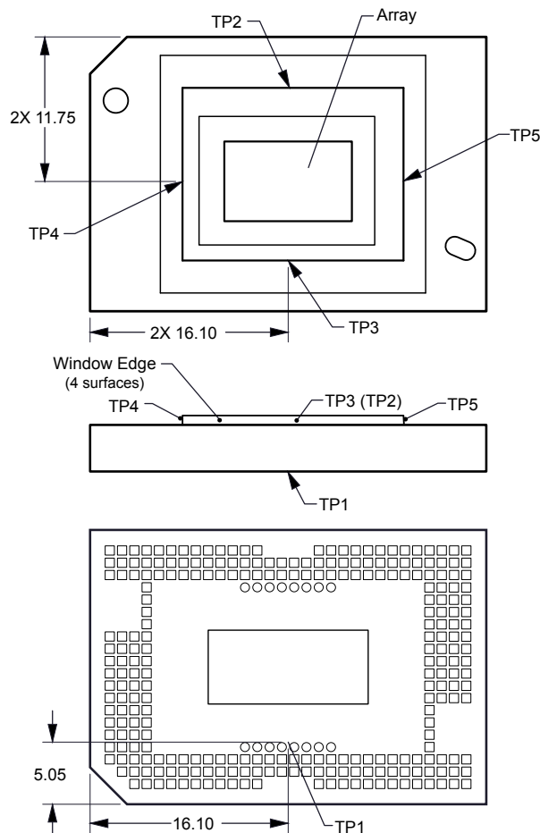
図 6-1. DMD Thermal Test Points
