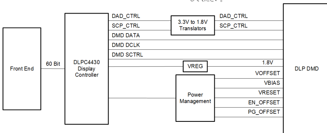
DLP480RE のアプリケーション概略図
